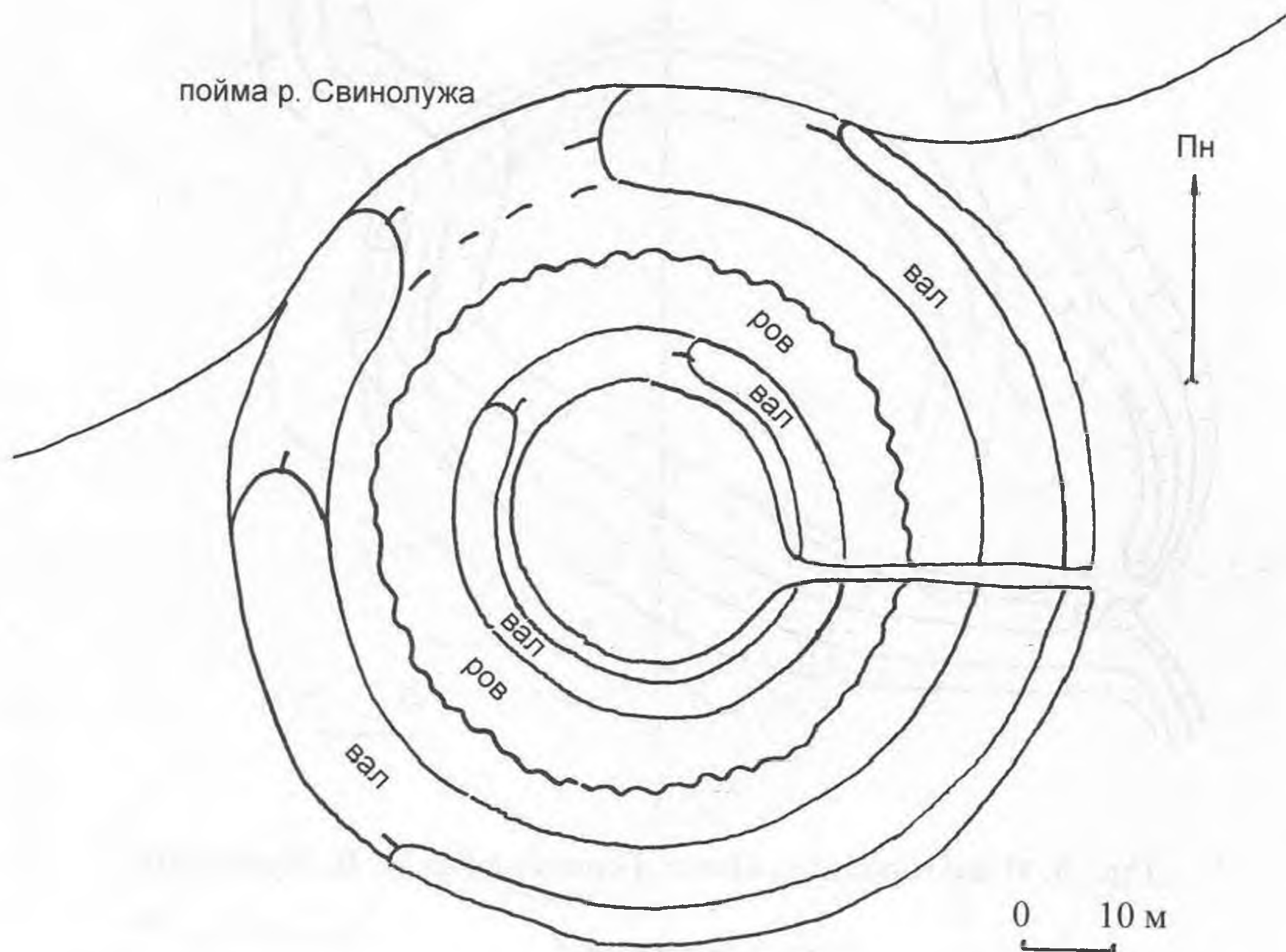
Рис. 7. План городища біля с. Городище на р. Свинолу́жжі (за М. П. Кучерою).
