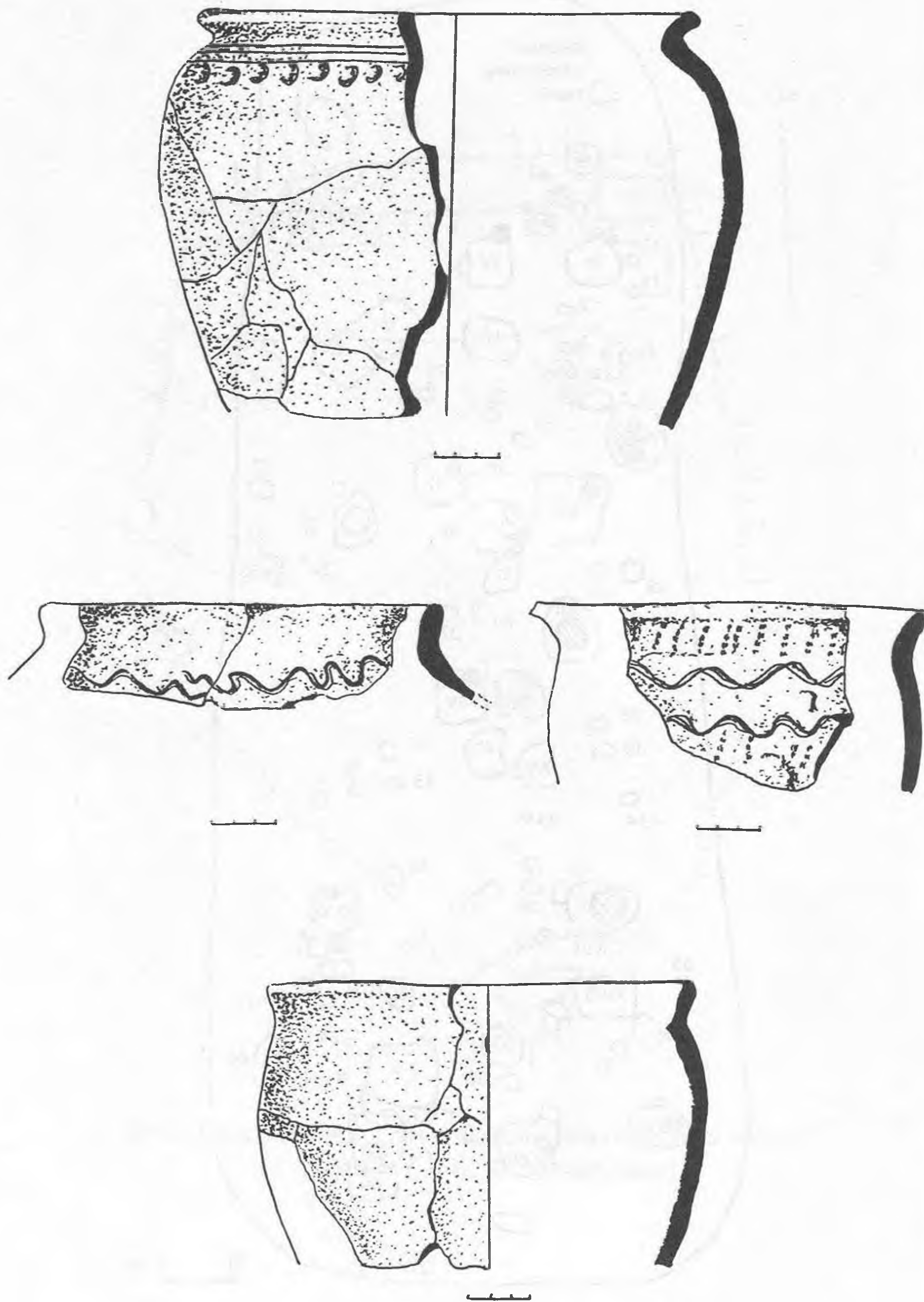
Рис. 11. Кераміка з об'єктів Малого Городського городища.
