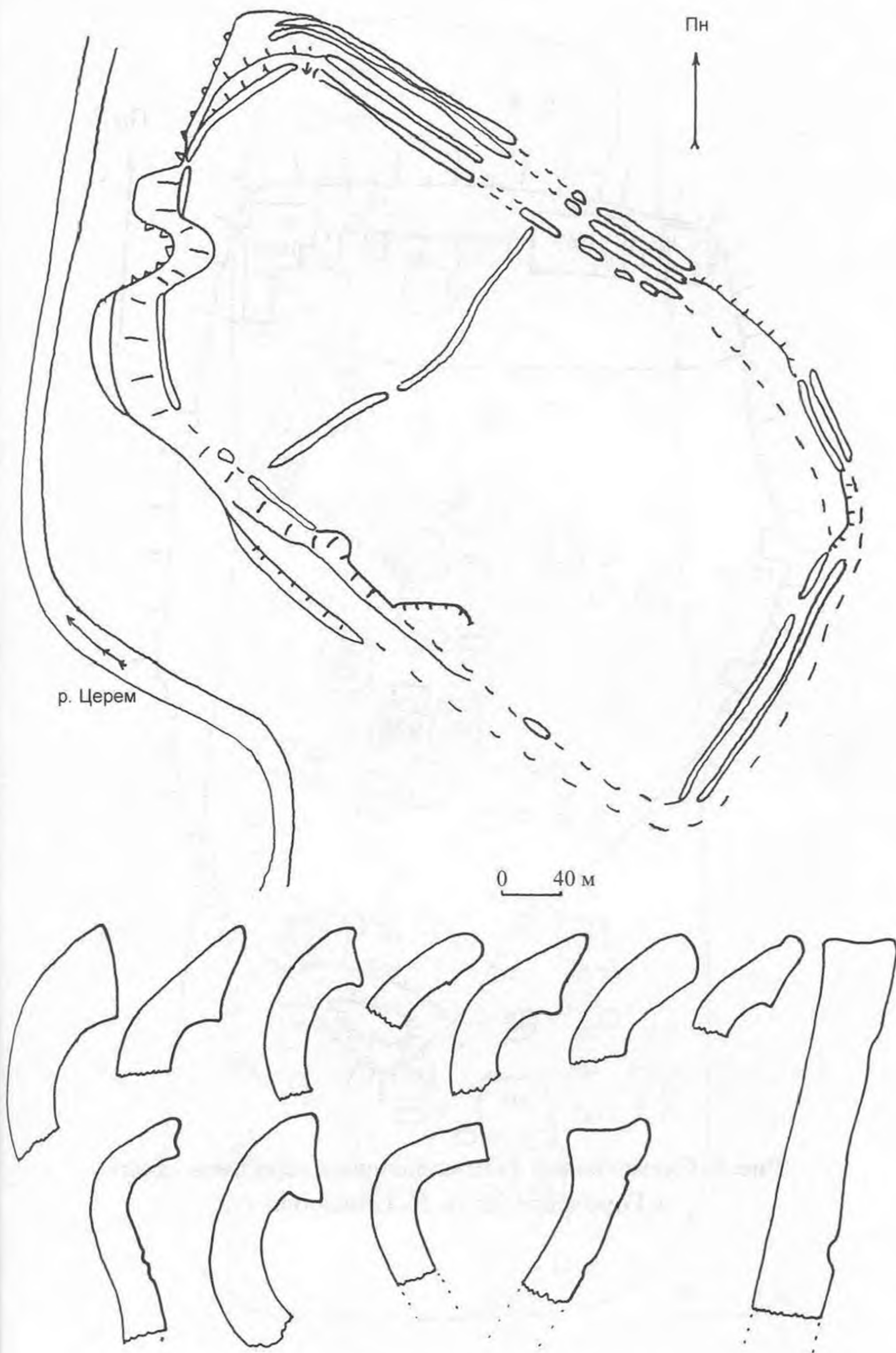
Рис. 8. План городища в с. Городище на р. Церем (за М. П. Кучерою) та профілі вінець кераміки з культурного шару.
