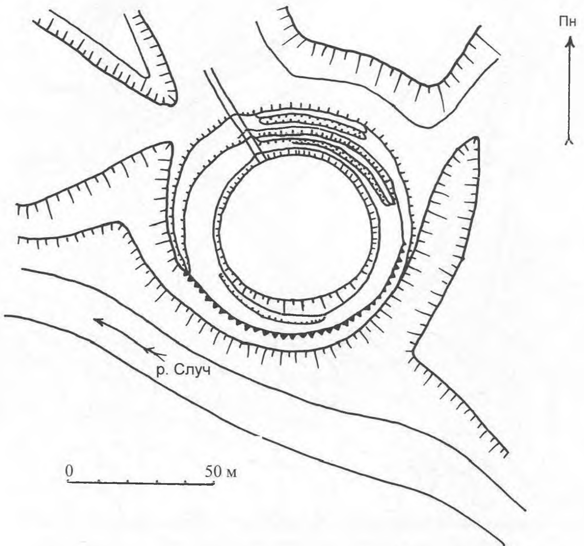
Рис. 39. План городища біля с. Миропіль (за М. П. Кучерою).
