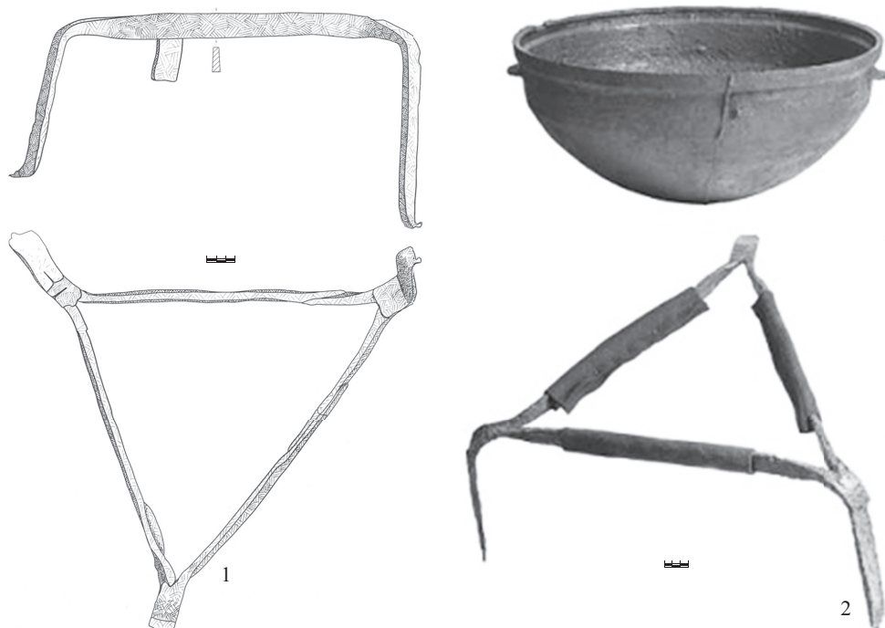
Рис. 3. Тагани: 1 – скарб на поселенні Котелівка 6; 2 – таган і казан з поселення Івченці
