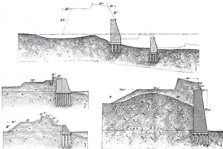
Рис. 5. Палі для ущільнення ґрунту під укріпленнями XVIII ст. за Ф. Ласковським: 1 – Смоленськ; 2 – Кронштадт 1753 р.; 3 – Кронштадт 1759 р.; 4 – Нейшлот
