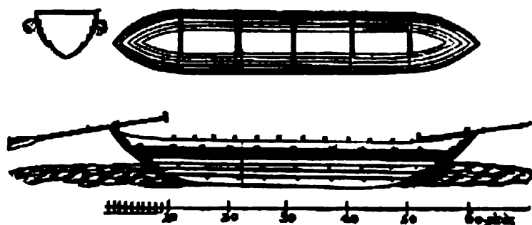
114. Чертеж казацкой «чайки» Гийома Левассера де Боплана в его книге «Description d'Ukraine» (Руан, 1660)
