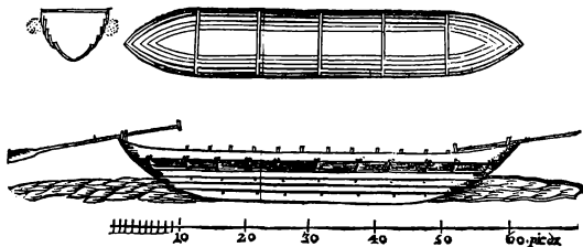
114. Кресленик козацької чайки Гійома Левасера де Боплана 1660 р.
