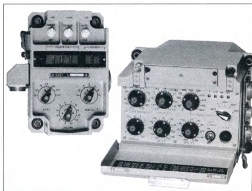
Балістичний обчислювач ЛІО-В
