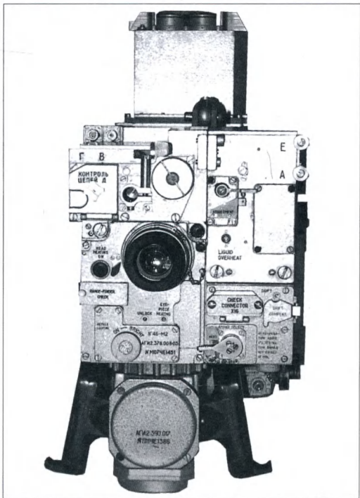
Приціл 1Г46М
