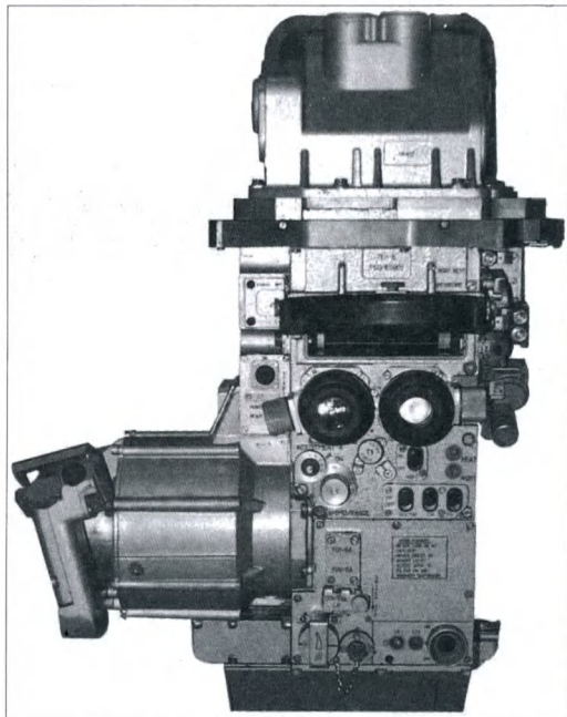
Приціл ТКН-5
