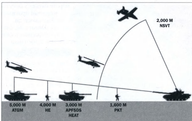
Дальність і радіус дії озброєння
