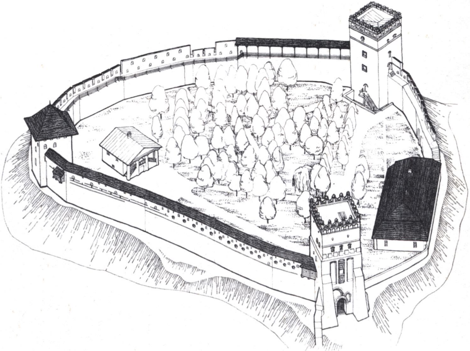
Замок після реставрації 60-70-х років — сьомого будівельного періоду. Аксонометрія (15,28)
