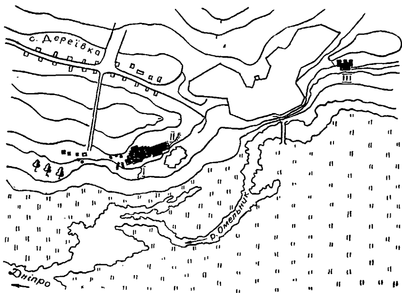
Рис. 13. Розташування поселення (I) та могильників II, III поблизу с. Деревки.
