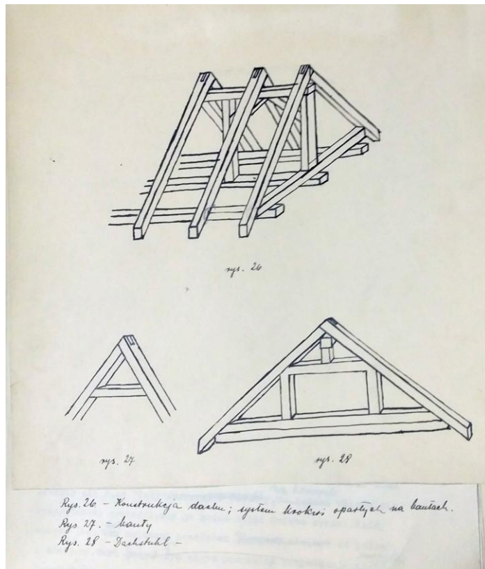
Конструкція даху
