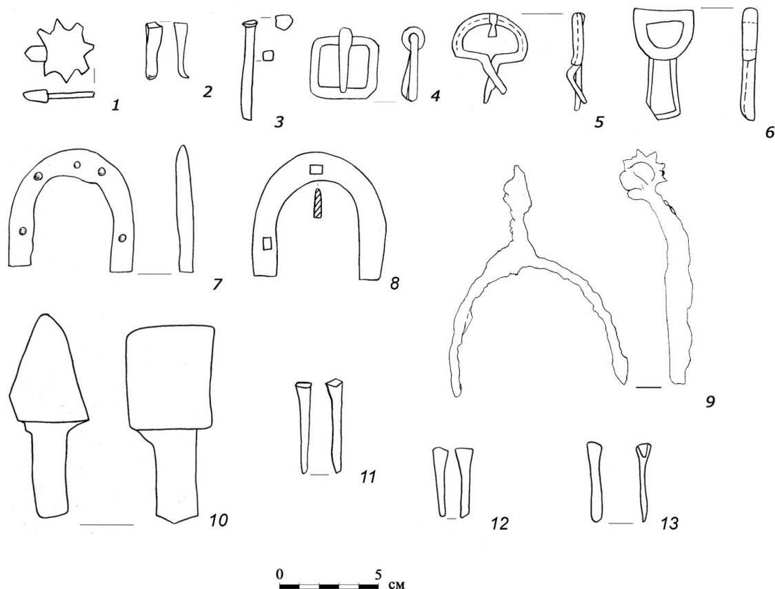
Рис. 7. Знахідки із розкопу I (1–5, 7–8, 10–13) та розкопу II (6, 9). 1 – фрагмент остроги; 2, 11–13 – вухналі; 3 – цвях; 4–5 – пряжки; 6 – фрагмент портупеї (?); 7–8 – підкови; 9 – острога; 10 – зубило Fig. 7. Materials from excavated area I (1–5, 7–8, 10–13) and excavated area II (6, 9). 1 – fragment of fish-fork; 2, 11–13 – wedges; 3 – nail; 4–5 – buckles; 6 – fragment of weapon-belt (?); 7–8 – horseshoes; 9 – fish-fork; 10 – chisel
