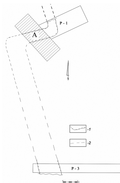
Рис. 6. Реконструкція фрагменту фортифікації табору. 1 – межі рову; 2 – реконструйована частина рову
