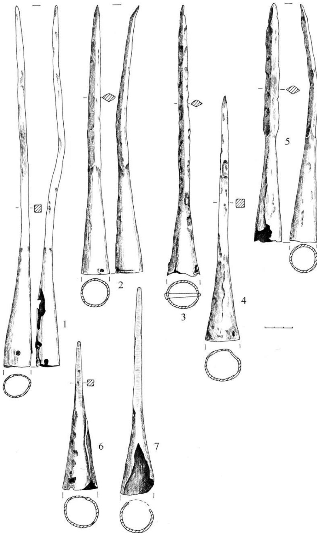
Рис. 9. Княжа Гора. Вістря списів. Залізо.
