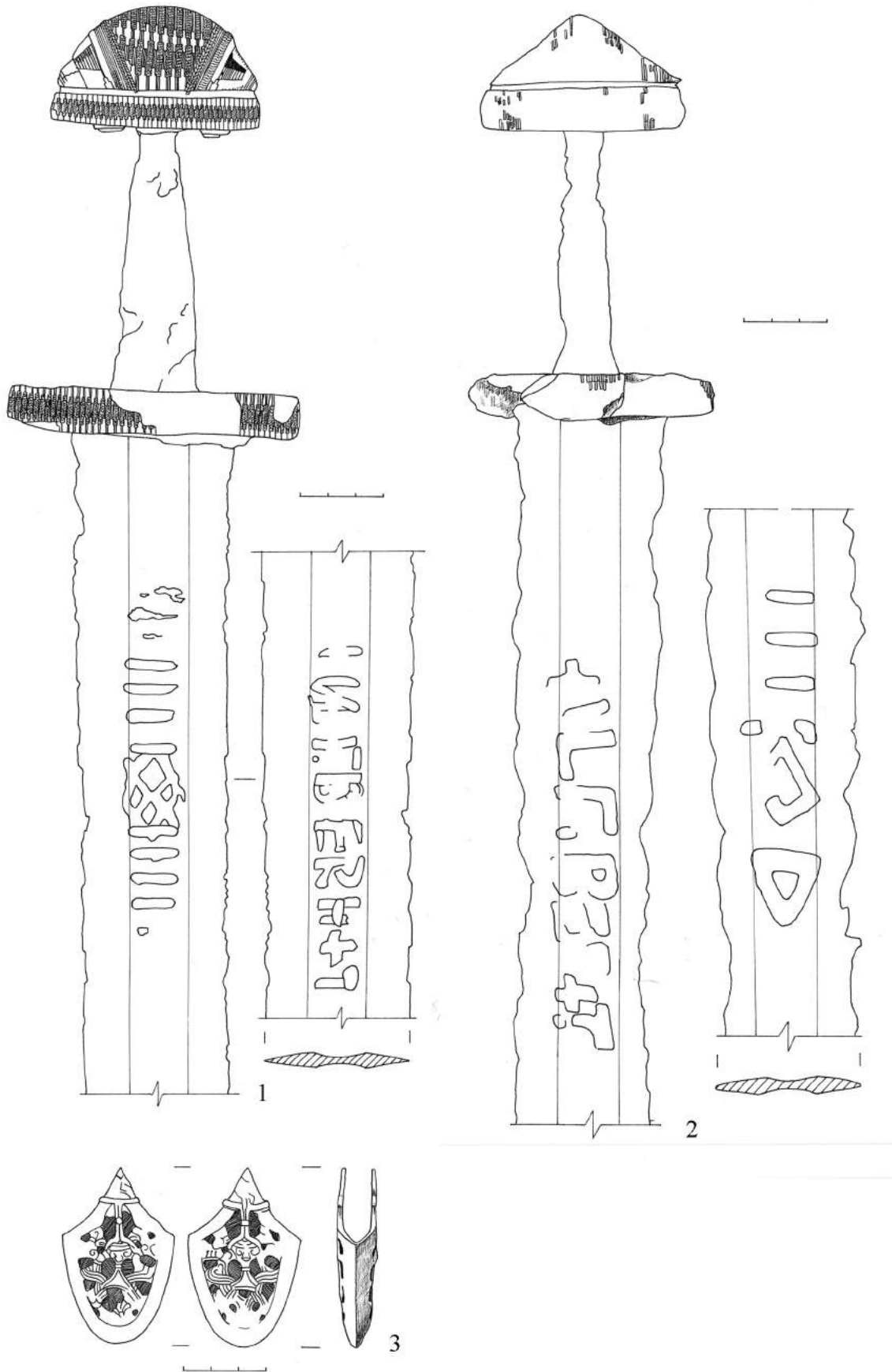
Рис. 39. Шестовицький могильник. Мечі та наконечник піхов. 1 – курган XXV (110), 2 – курган II (36); 3 – курган X (42). 1, 2 – залізо, срібло; 3 – бронза.
