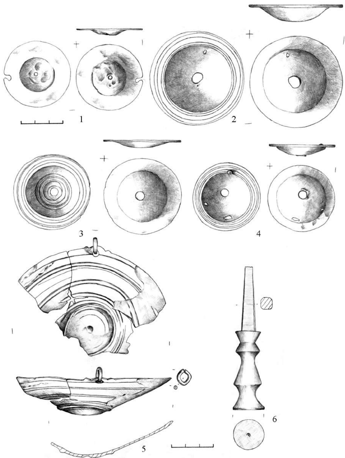
Рис. 28. Княжа Гора. Свічники та лампада. Бронза.
