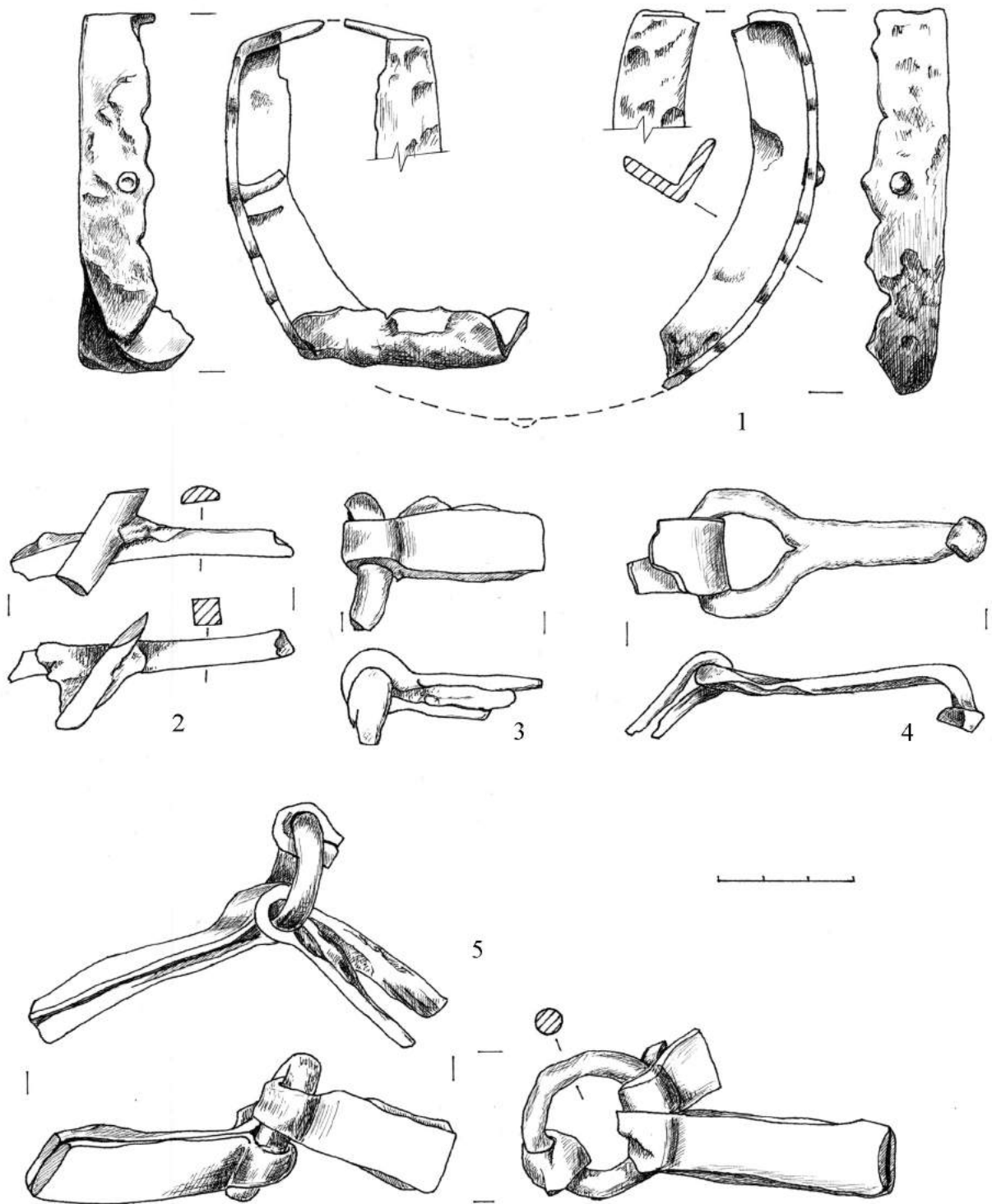
Рис. 46. Шестовицький могильник. Деталі сагайдака. Курган XXV (110). Залізо.
