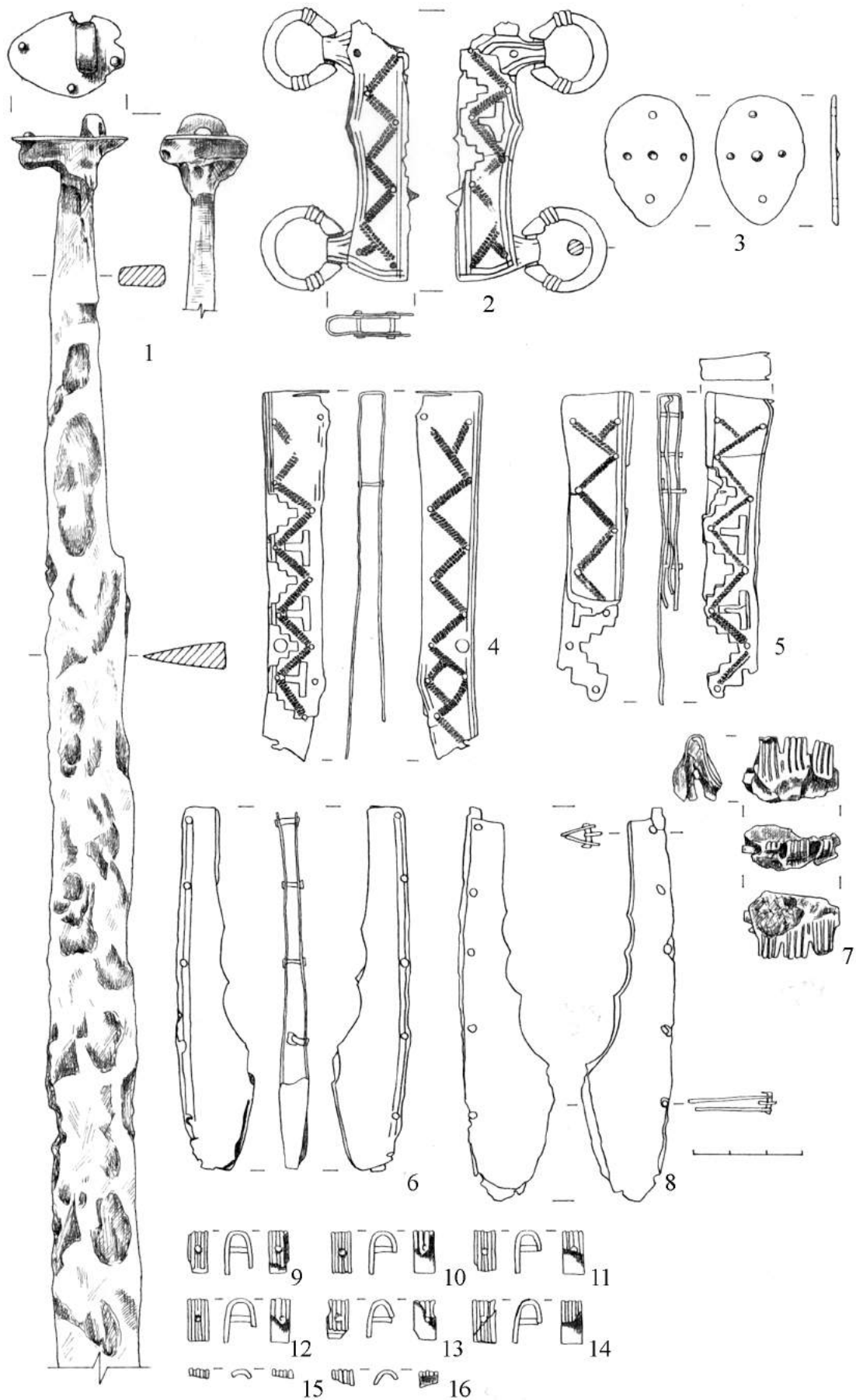
Рис. 48. Шестовицький могильник. Скромасакс і деталі піхов. 1-4, 7-16 – курган XII (145); 5, 6 – курган XXIV (30).
