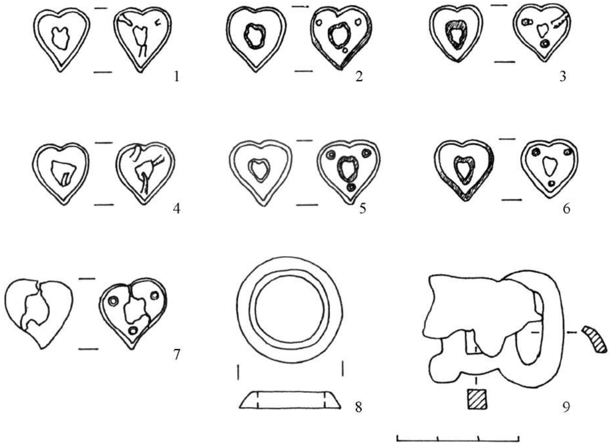
Рис. 1. Табайвський могильник. Матеріали з розкопок кургану першої групи 1904 р. Бронза.
