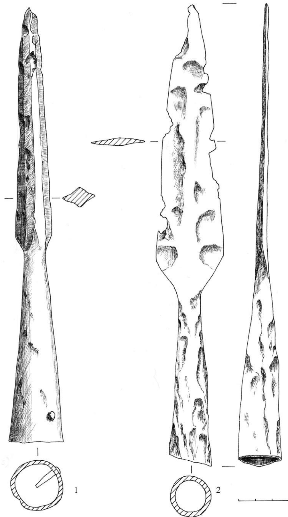
Рис. 38. Шестовицький могильник. Вістря списів. 1 – курган XII (145); 2 – курган II (36). Залізо.
