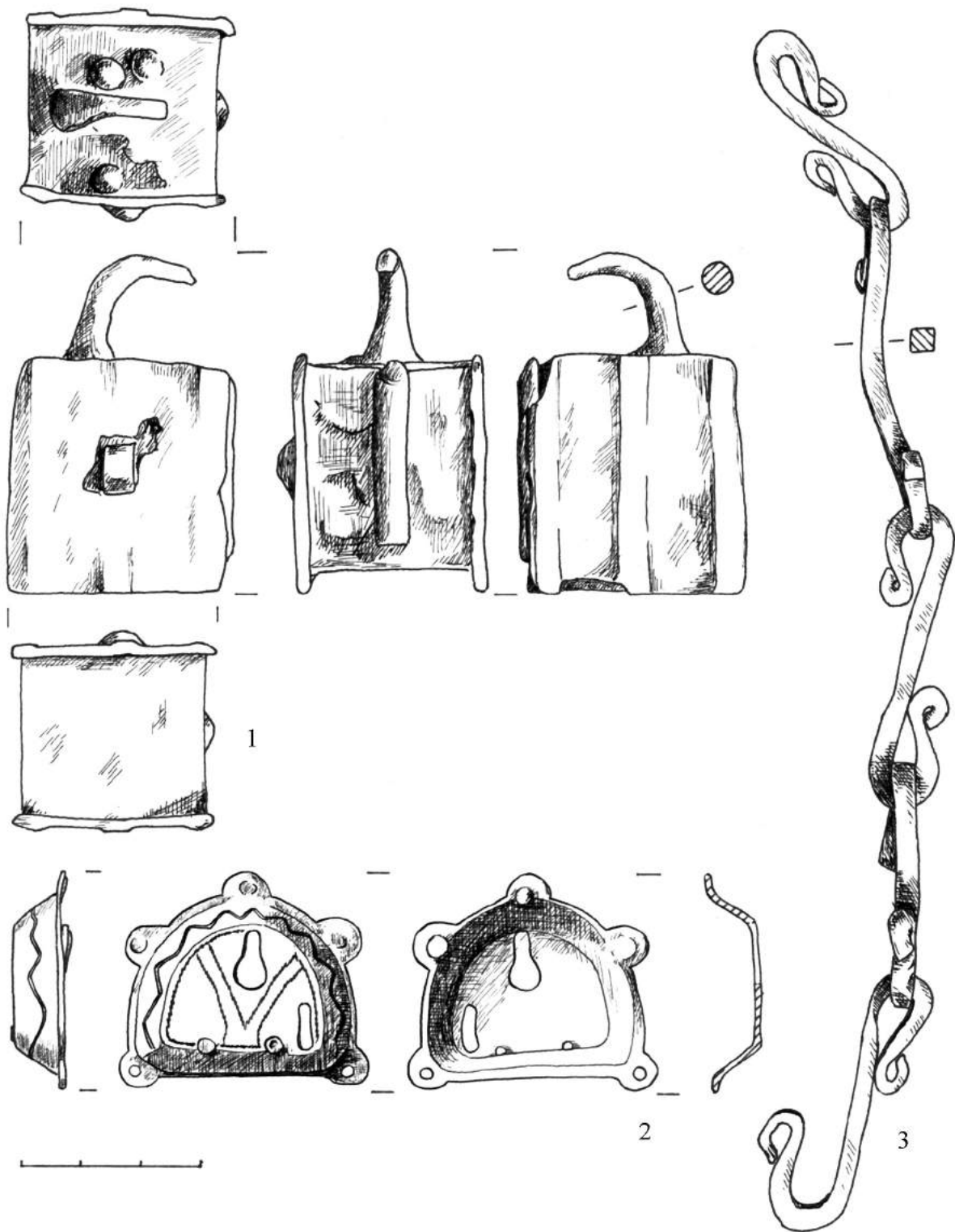
Рис. 23. Княжа Гора. Побутові речі. 1, 3 – залізо; 2 – бронза.
