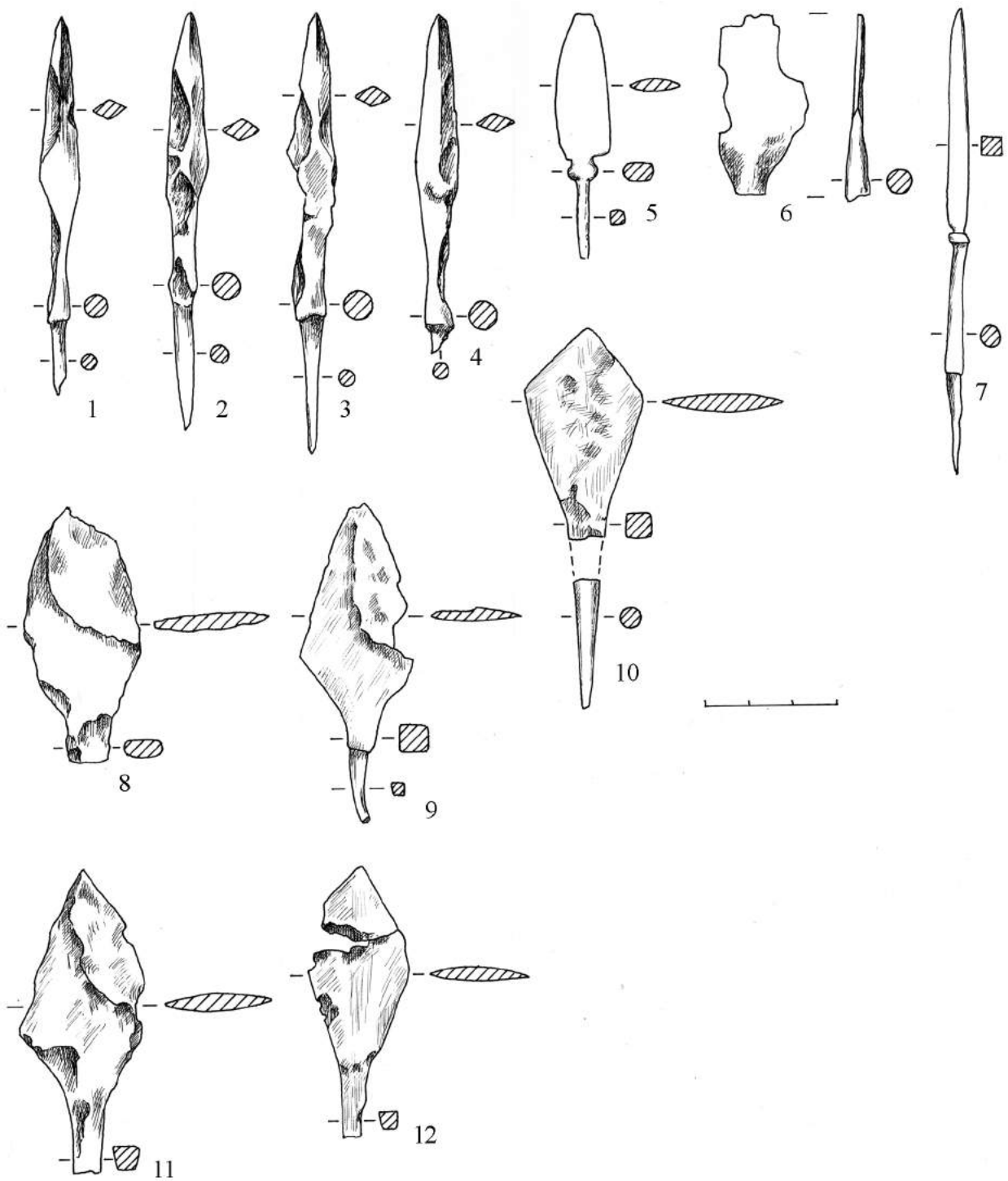
Рис. 33. Шостовицький могильник. Вістря стріл. Залізо.
