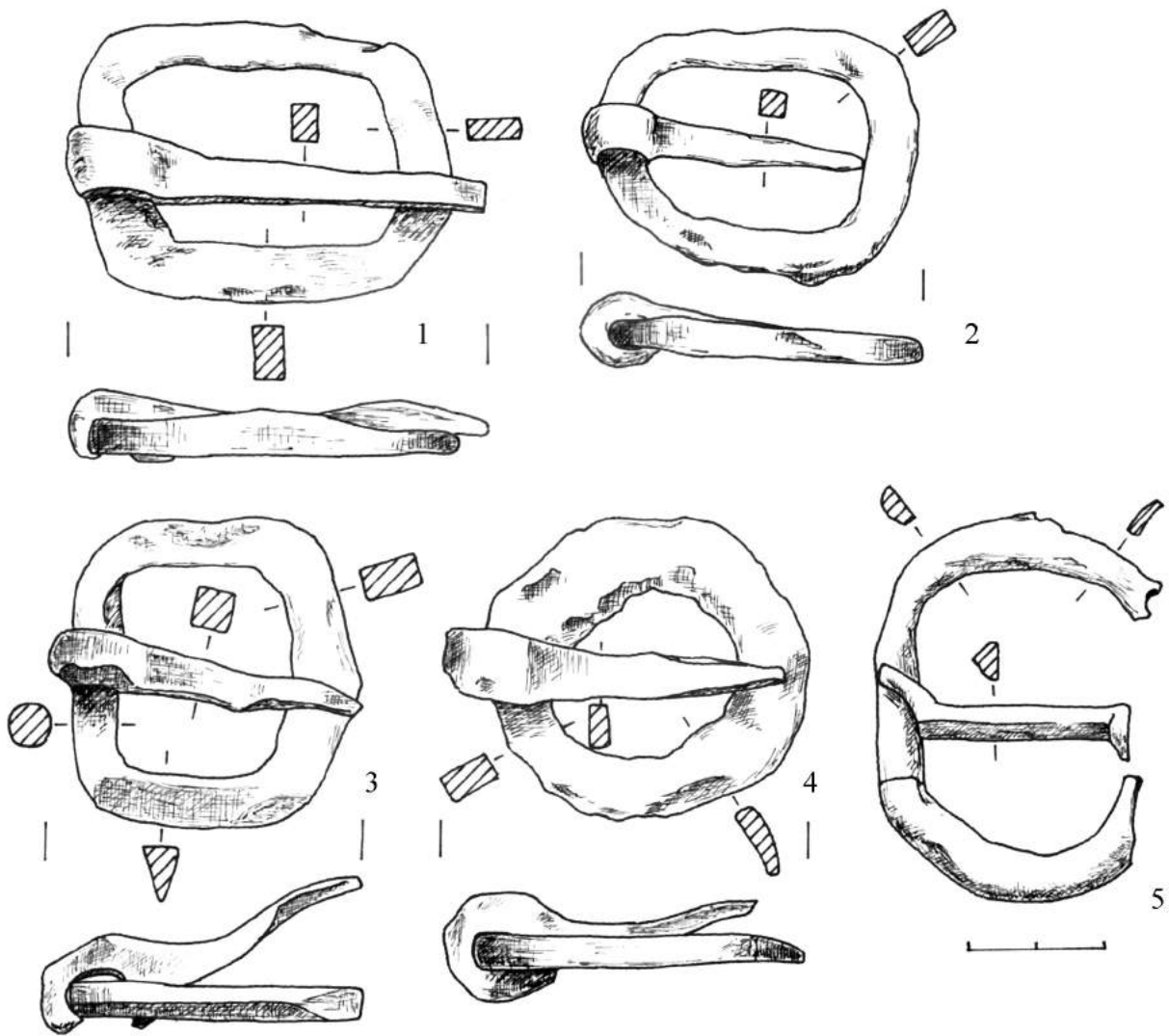
Рис. 44. Шестовицький могильник. Пряжки. 1 – курган X (42); 2, 5 – курган XXV (110); 3 – курган XII (145); 4 – курган XII (145). Залізо.
