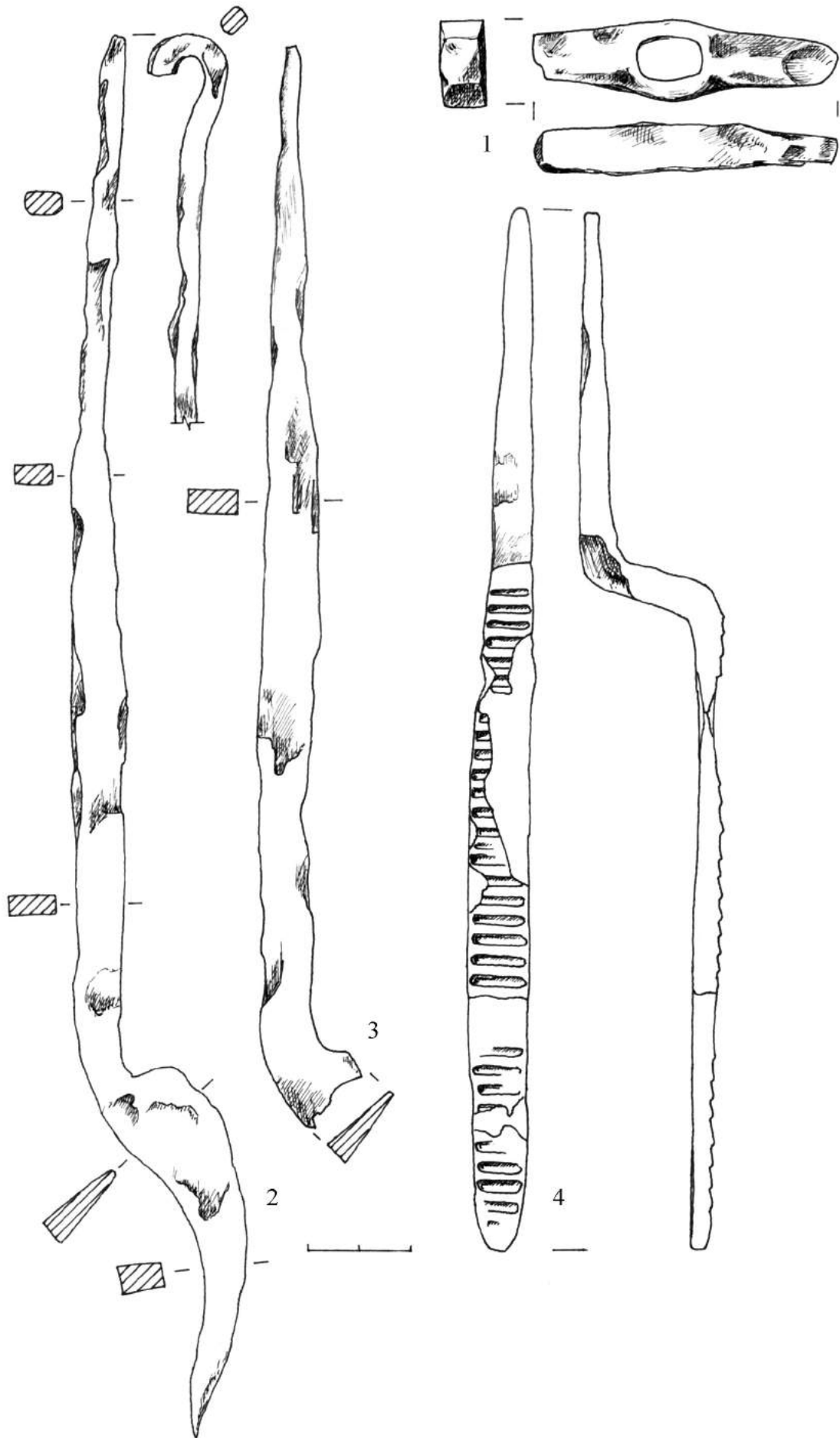
Рис. 37. Знаряддя праці. Курган II (36). Залізо.
