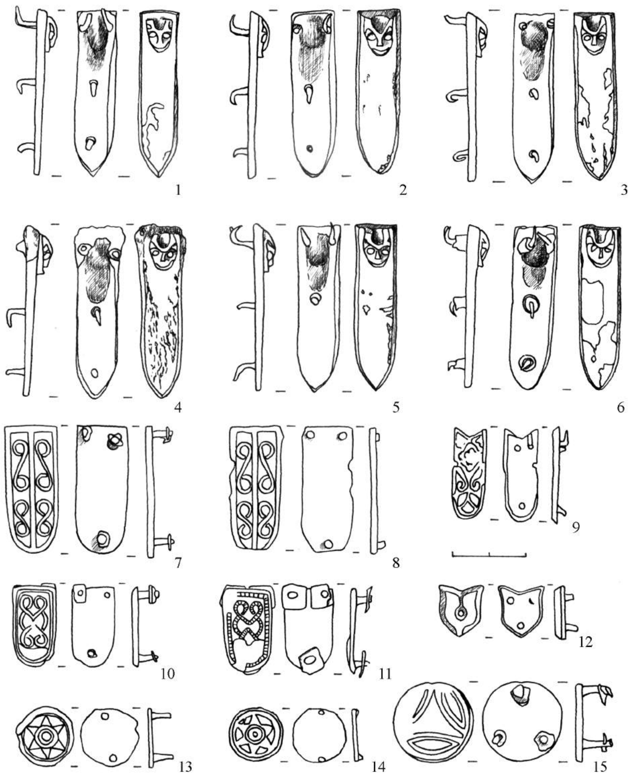
Рис. 43. Шестовицький могильник. Ременні прикраси. 1–6, 12 – курган X (42); 7–9 – курган IX (31); 10, 11, 13, 14 – курган XXII (93); 15 – курган I (18). Бронза.
