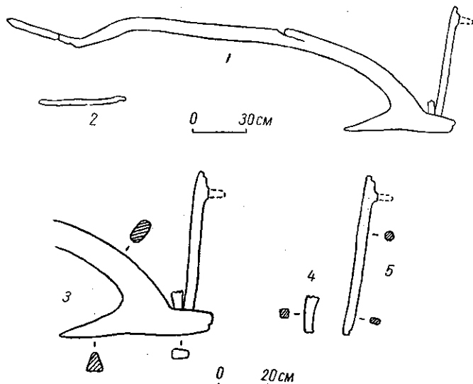
Рис. 5. Рало бронзового віку з с. Полісся:
