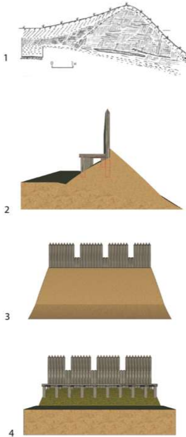
Рис. Г.1. Городище Грушвиця (земляний відкіс з гостроколом та галереєю з внутрішнього боку): перерізи оборонного валу (1) [Прищеп, 2016. Рис. 103] й оборонної лінії (2); реконструкція оборонної лінії – вигляд спереду (3) і з внутрішнього боку (4). [Креслення виготовлені автором]
