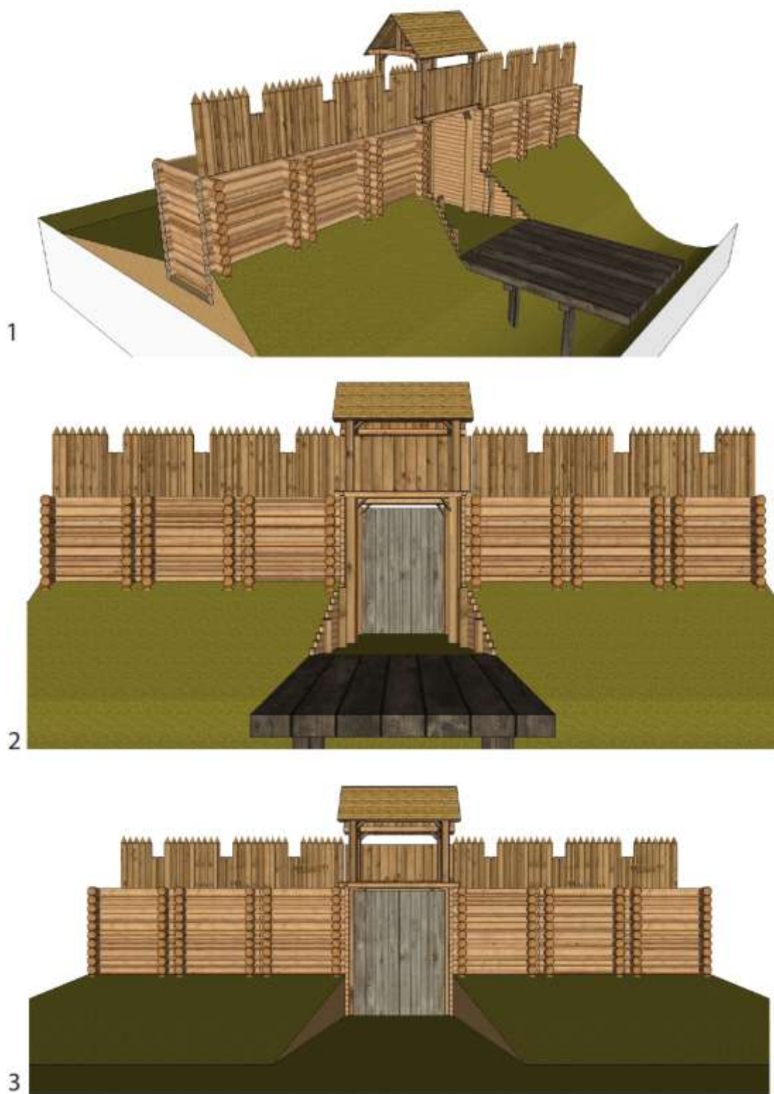
Рис. Г.6. Городище Коростень ІІІ (заповнені землею городні з надбудовою-гостроколом та в'їздом каркасно-стовпової конструкції): гіпотетичні реконструкції оборонної лінії (1) і проїзду через неї (2); вигляд на оборонну лінію з внутрішнього боку (3). [Креслення виготовлені автором]
