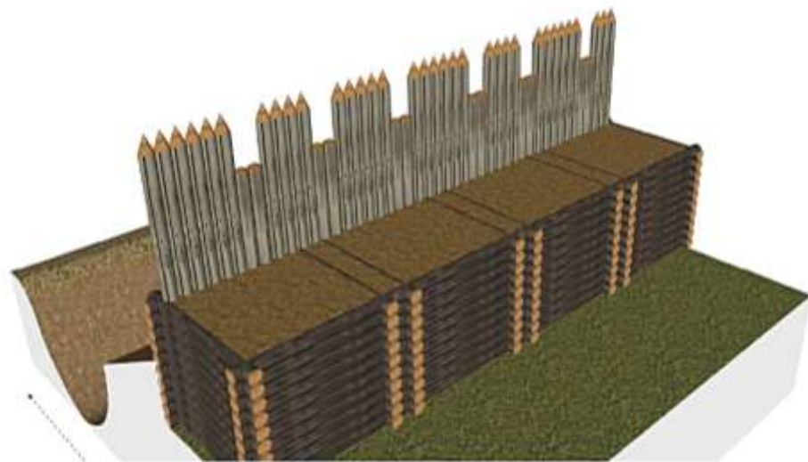
Рис. Г.8. Городище Маморниця (заповнені землею городні з гостроколом-надбудовою ): гіпотетична реконструкція оборонного валу – вигляд з зовнішнього боку (1); гіпотетична реконструкція бойової галереї (2). [Креслення виготовлені автором]
