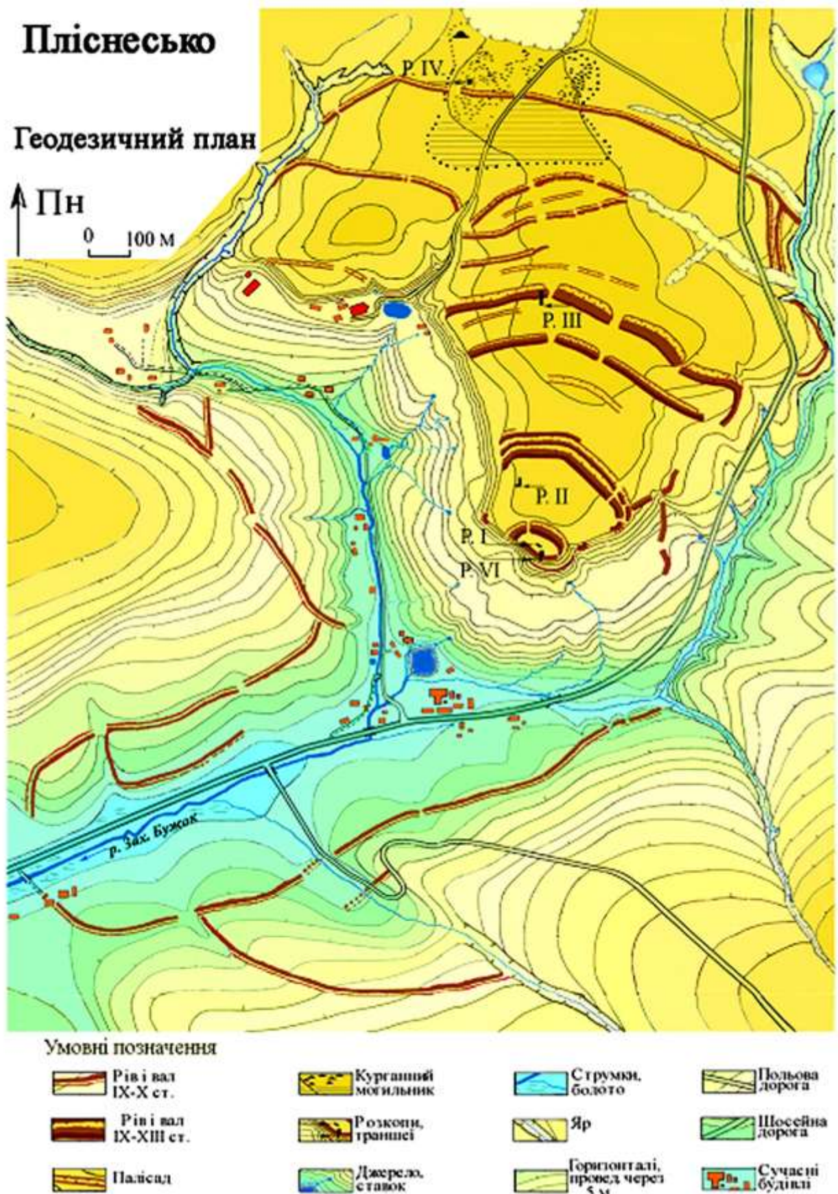
Рис. В.32. План Пліснеського городища (IV тип) [Филипчук, 2012. Карта 6].
