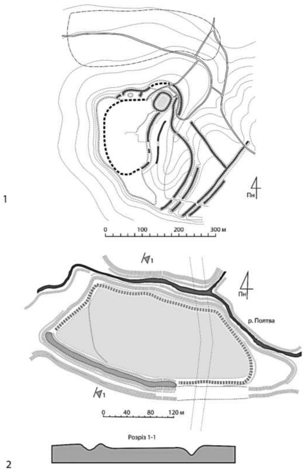
Рис. В. 29. Плани городищ IV типу: Жорнів (1), (план опрацьований автором на основі матеріалів виготовлених Б. Прищепою [Прищеп, 2016. Рис. 104]) і Буськ (2) (план та профіль опрацьований автором на основі матеріалів виготовлених П. Раппопорт [Раппопорт, 1967. Рис. 37]).
