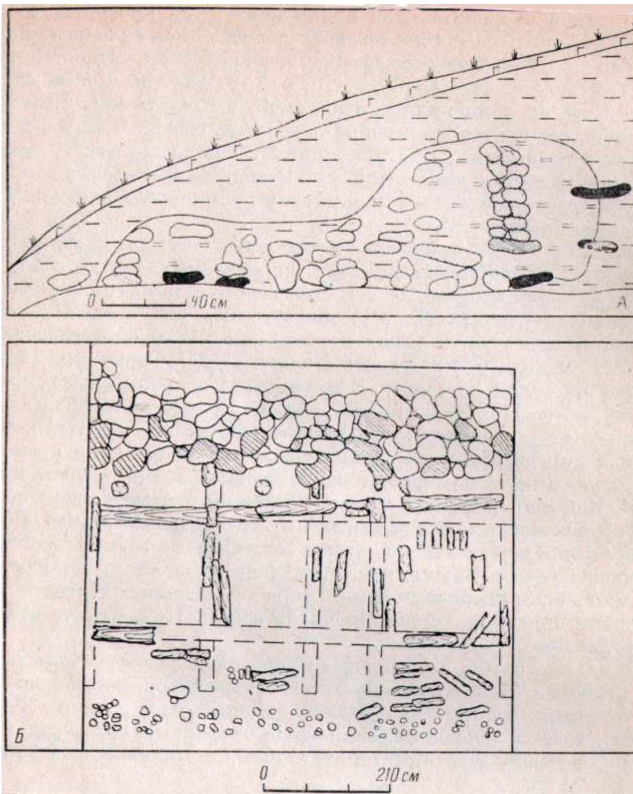
Рис. Г.11. Переріз валу (А) і план оборонної фортифікації (Б) городища Ревне ІБ [Тимошук, 1990. Рис. 24]. [Креслення виготовлені автором]
