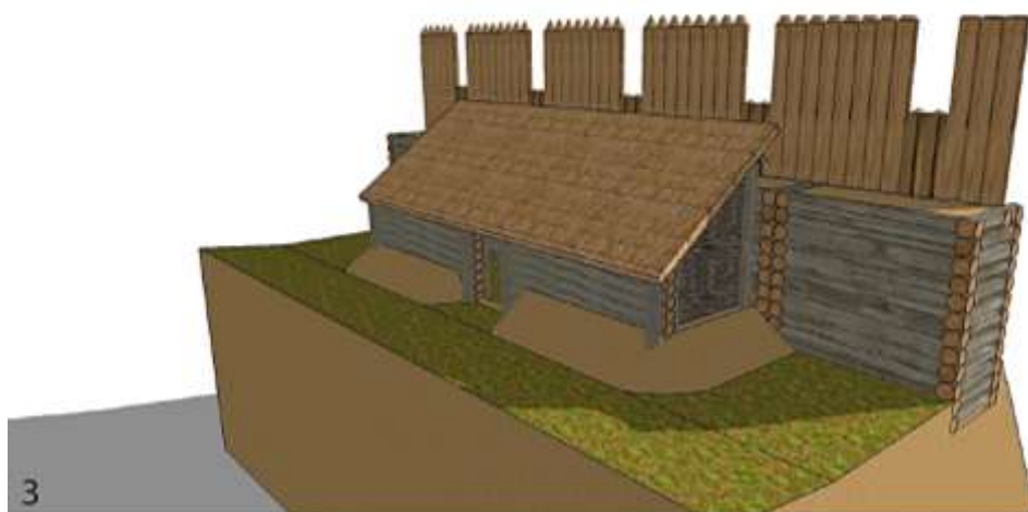
Рис. Г.9. Городище Мотич (заповнені землею городні з гостроколом-надбудовою та з наземною спорудою, що прилягає до оборонні стіни з внутрішнього): гіпотетична реконструкція оборонної лінії (1); надбудова у вигляді гостроколу з бійницями (2); наземна прибудова з внутрішнього боку (3). [Креслення виготовлені автором]
