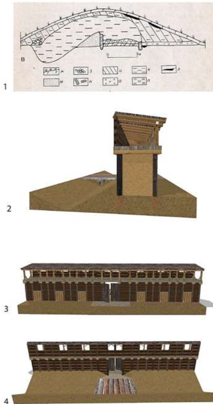
Рис. Г.7. Городище Ломачинці (дві каркасно-стовпові стіни, що формують стійково-балкову конструкцію з критою бойовою галереєю на другому ярусі): переріз оборонного валу (1) [Тимощук, 1990. Рис. 12]; переріз оборонної лінії (2); гіпотетична реконструкція фортифікації – вигляд з внутрішнього (3) і зовнішнього (4) боку. [Креслення виготовлені автором]
