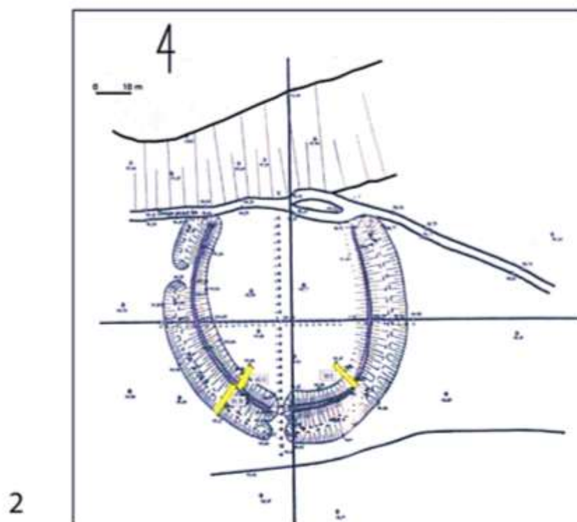
Рис. В.1. Плани городищ I типу: Каніє (1) [Cichomski J., 1980. Rys. 8] і Бусинець (2) [Cichomski J., 1980. Rys. 15].
