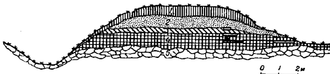
Рис. 6. Городище III. Розріз валу на східному краю (1934 р.): 1 — світло-жовтий пісок; 2 — темно-сірий пісок; 3 — світлий глиняно-піщаний шар; 4 — темний глиняно-піщаний шар; 5 — граніт.
