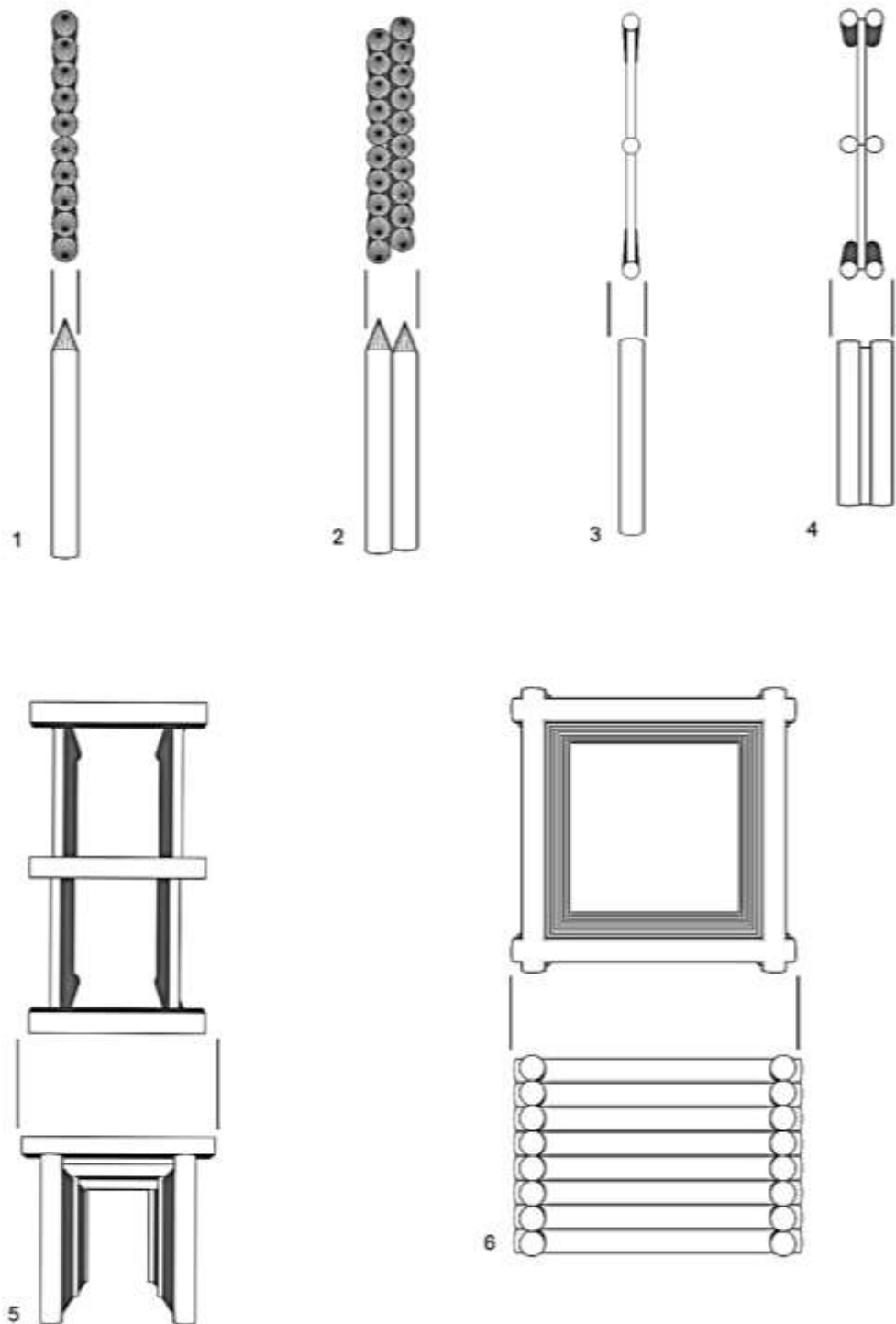
Рис. Е.1. Типові конструкції фортифікацій:.. однорядний гострокіл (1); дворядний гострокіл (2); каркасно-стовпова конструкція (3); каркасно-стовпова конструкція з подвійними вертикальними стояками (4); подвійна каркасно-стовпова конструкція з галереєю зверху (5); городні (6). [Схема виготовлена автором]
