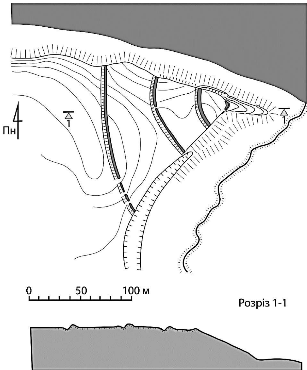
Рис. В1.3. План городища (II типу) Копачинці (план та профіль опрацьований автором на основі матеріалів виготовлених Б. Томенчуком [Томенчук, 2008. Рис. 307]).
