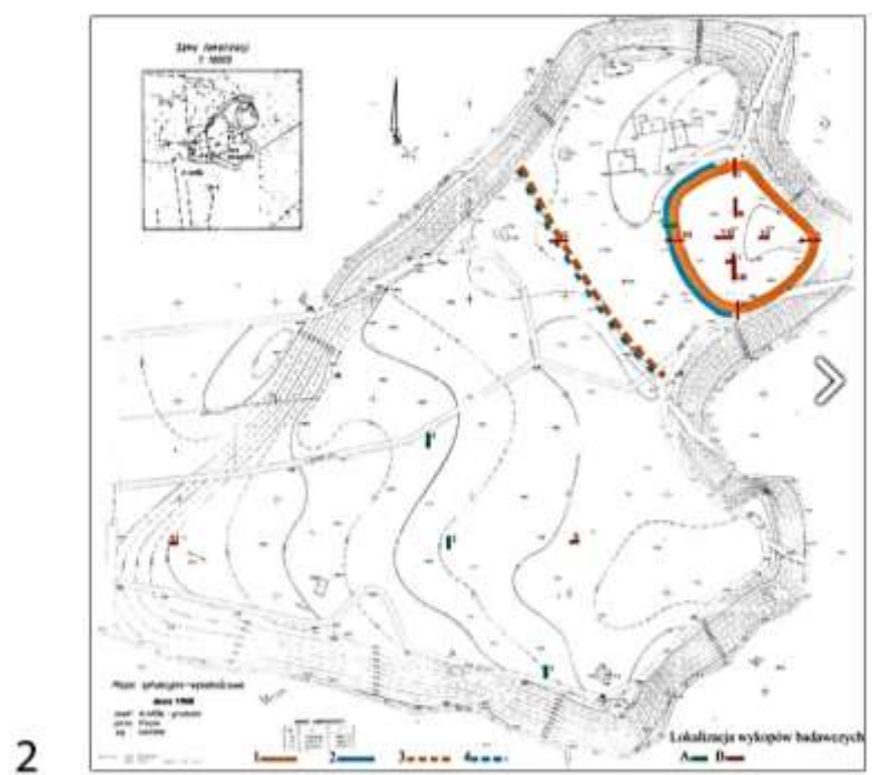
Рис. В.16. Плани городищ III типу: Грабув (1) [Mączka G., 2017, Rys. 5] та Кларув (2) [Włodarczyk D., 2002. Rys. 2].
