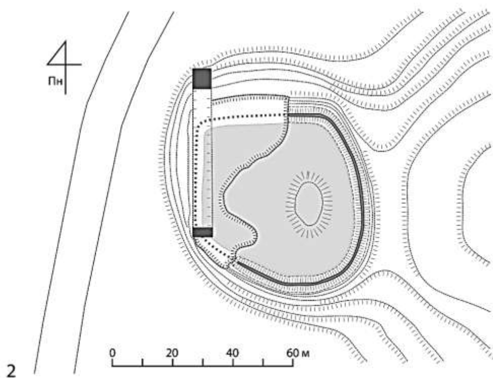
Рис. В.22. Плани городищ III типу: Несолонь (1), (план опрацьований автором на основі матеріалів виготовлених Б. Звіздецьким [Звіздецький, 2008. Рис. 46]). і Грушвиця Перша (2), (план опрацьований автором на основі матеріалів виготовлених Б. Прищепи [Прищепи, 2016. Рис. 103])..
