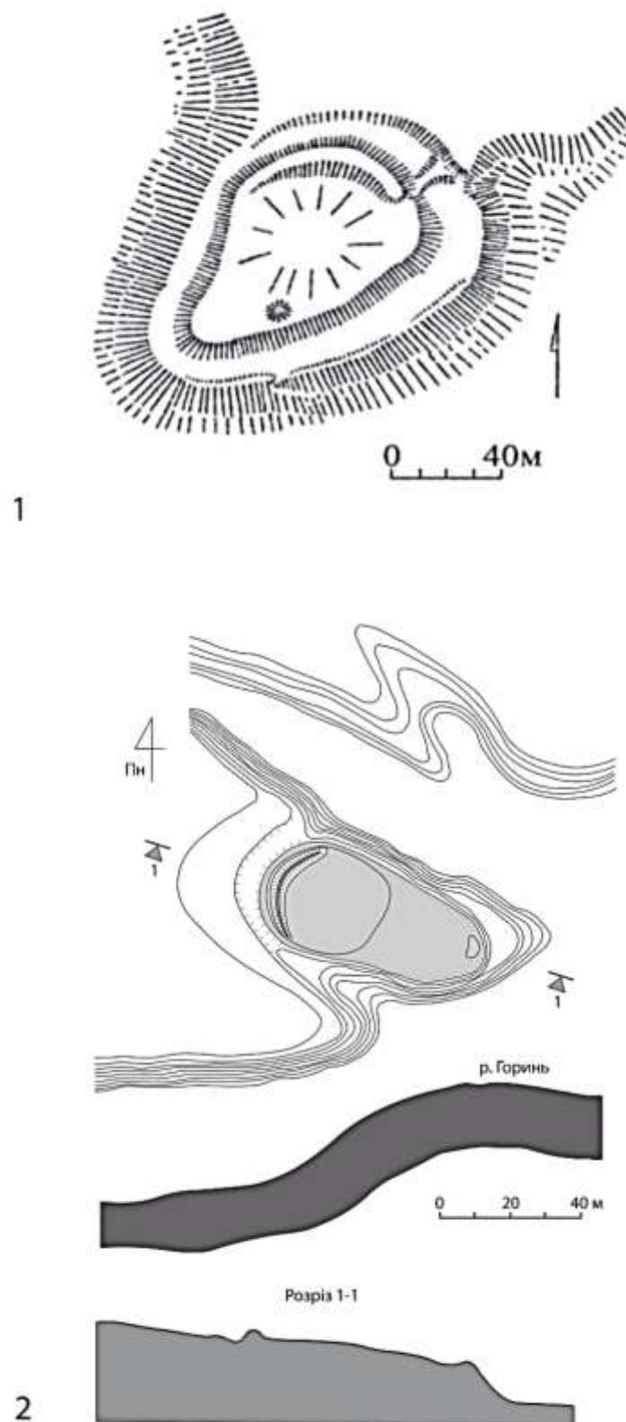
Рис. В.11. Плани городищ II типу: Стеблівка (1) [Прищеп, 2016. Рис. 5] та Бичаль (2) (план та профіль опрацьований автором на основі матеріалів виготовлених Б. Прищепою [Прищеп, 2016. Рис. 13]).
