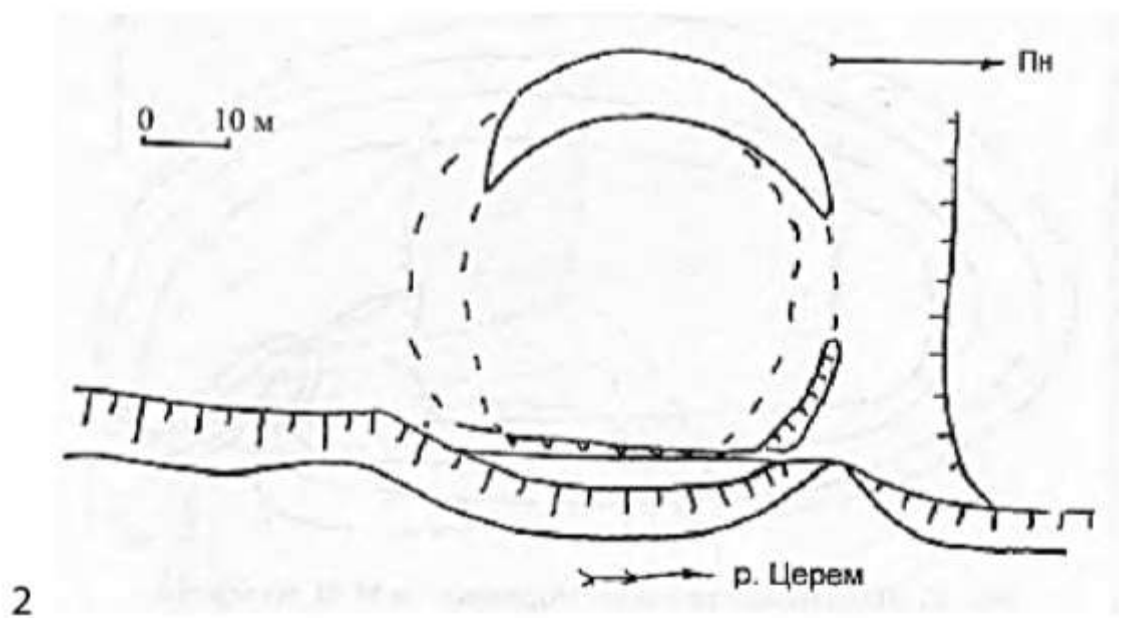
Рис. В.7. Плани городищ І типу: Затурці (1) [Раппопорт, 1967. Рис. 28].та Пилиповичі (2) [Звіздецький, 2008. Рис. 49].
