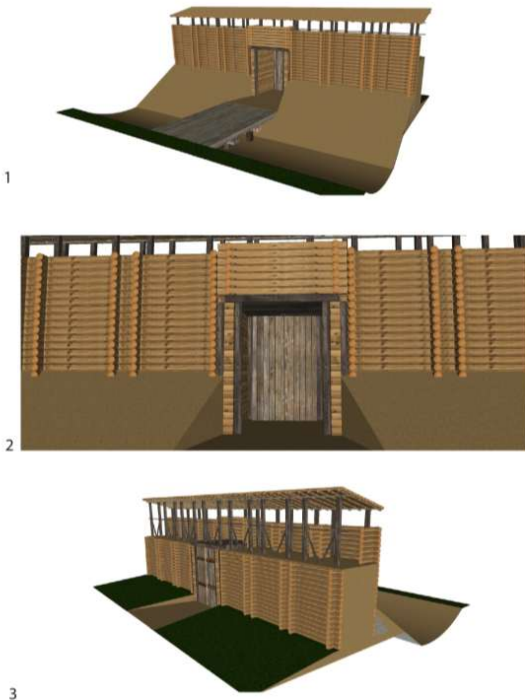
Рис. Г.12. Городище Ревне ІБ (заповнені землею городні з дахом над бойовою галереєю та каркасно-стовповою конструкцією в'їзду): гіпотетична реконструкція головної оборонної лінії (1); конструкція в'їзду на укріплений майдан (2); імовірний вигляд на фортифікацію з внутрішнього боку (3). [Креслення виготовлені автором]
