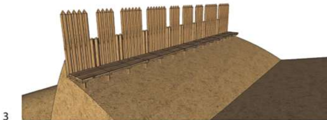
Рис. Г.3. Жорнівське городище (земляний відкіс з гостроколом та галерією з внутрішнього боку): переріз зовнішнього оборонного валу (1) [Прищеп, 2016. Рис. 105]; переріз того ж валу, відтворений за допомогою програми для 3D моделювання SketchUp(2); гіпотетична реконструкція оборонного валу (3). [Креслення виготовлені автором]
