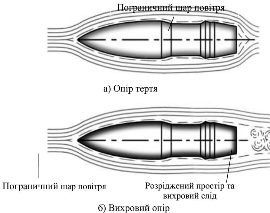
Рисунок 2.3 – Походження сили опору повітря внаслідок тертя та вихрового опору
