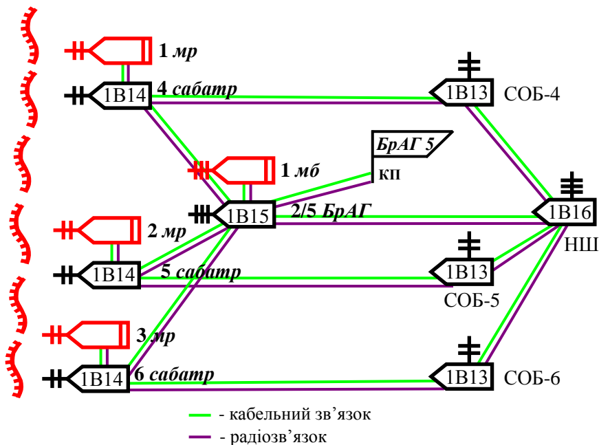
Рисунок 10.4 – Схема радіозв'язку артилерійського дивізіону (варіант)
