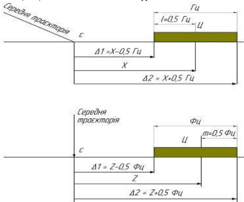
Рисунок 3.17 – Віддалення ЦРС відносно центра цілі
