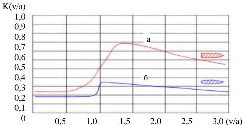
Рисунок 2.7 – Графік функції : а – снаряд з циліндричною запаясковою частиною (стара фугасна граната); б – довгастий снаряд із конічною запаясковою частиною
