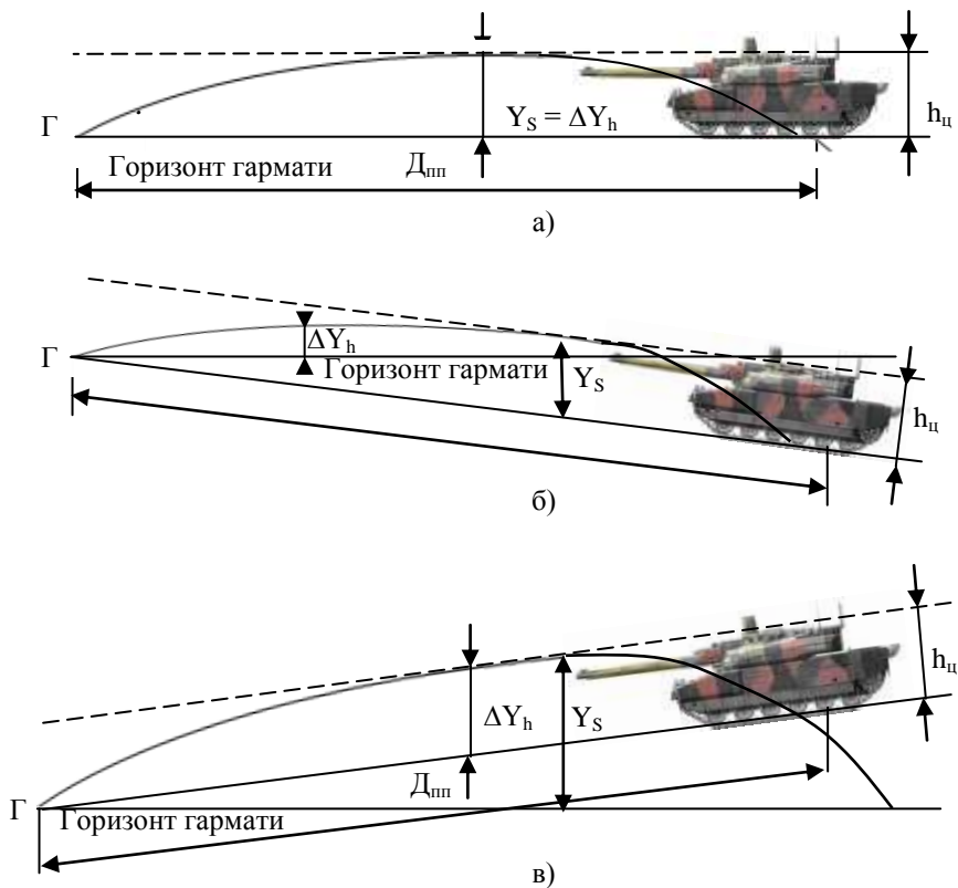
Рисунок 12.1 – Сутність дальності прямого пострілу: а) ціль на горизонті гармати; б) ціль вище горизонту гармати; в) ціль нижче горизонту гармати
