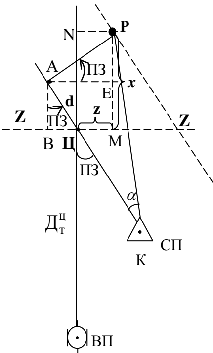
Рисунок 8.2 – Виведення формул для аналітичного розрахунку коректур
