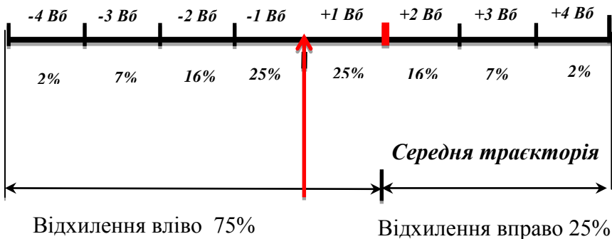
Рисунок 3.9 – Шкала розсіювання
