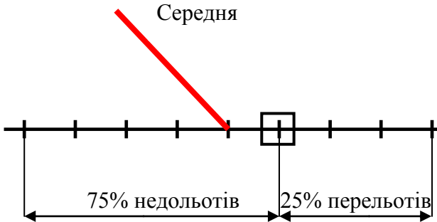
Рисунок 3.8 – Шкала розсіювання
