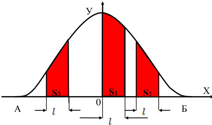
Рисунок 3.2 – Закон розсіювання
