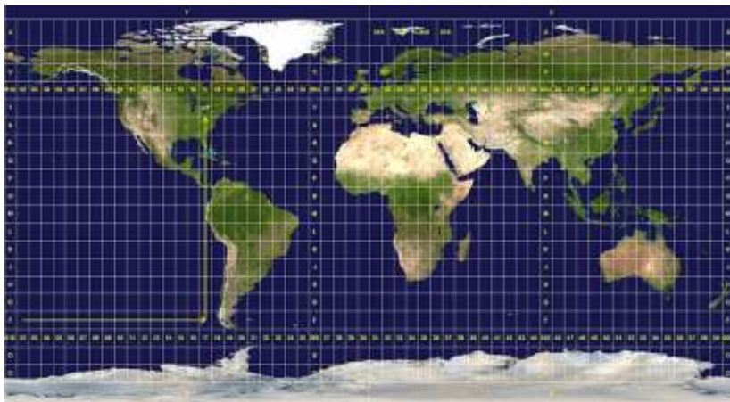
Рисунок 15.1 – Зони UTM
