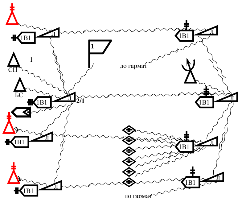
Рисунок 10.5 – Схема кабельного зв'язку артилерійського дивізіону (варіант)
