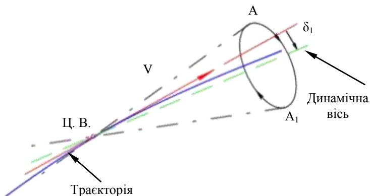
Рисунок 2.9 – Повільний конічний рух осі снаряда за криволінійною траєкторією: Ц. В. – центр ваги снаряда; \delta_1 – кут відхилення динамічної осі від дотичної (за правою нарізкою – вправо від точки кидання)
