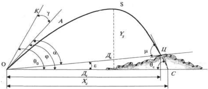
Рисунок 2.1 – Елементи траєкторії:
