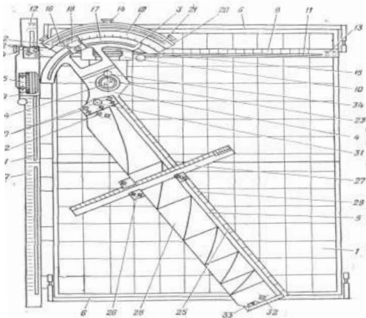
Рисунок 5.7 – Загальний вигляд приладу ПУВ-9:
