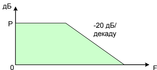
Рисунок 2.11 Характеристика передавання фазового тремтіння (відповідно до рекомендації ITU рис. 4/G.984.2)
