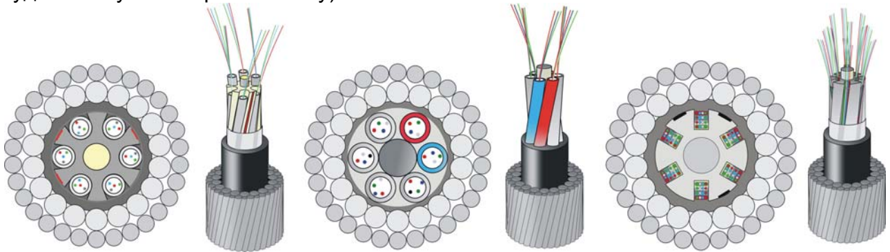
Рисунок 3.5 Конструкція кабелю, вбудованого в грозозахисний трос
