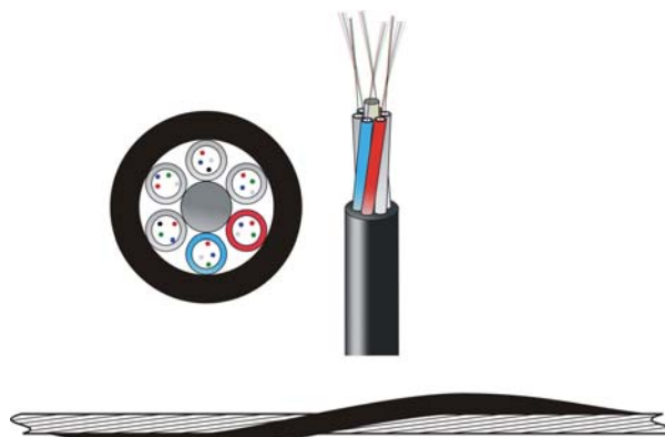
Рисунок 3.7 Конструкція навивного кабелю
