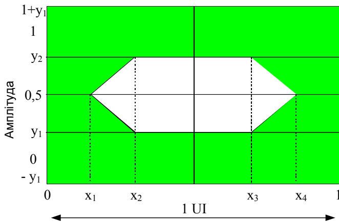
Рисунок 2.4 Око-діаграма для низхідного потоку (відповідно до рекомендації ITU рис. 6/G.983.1)
