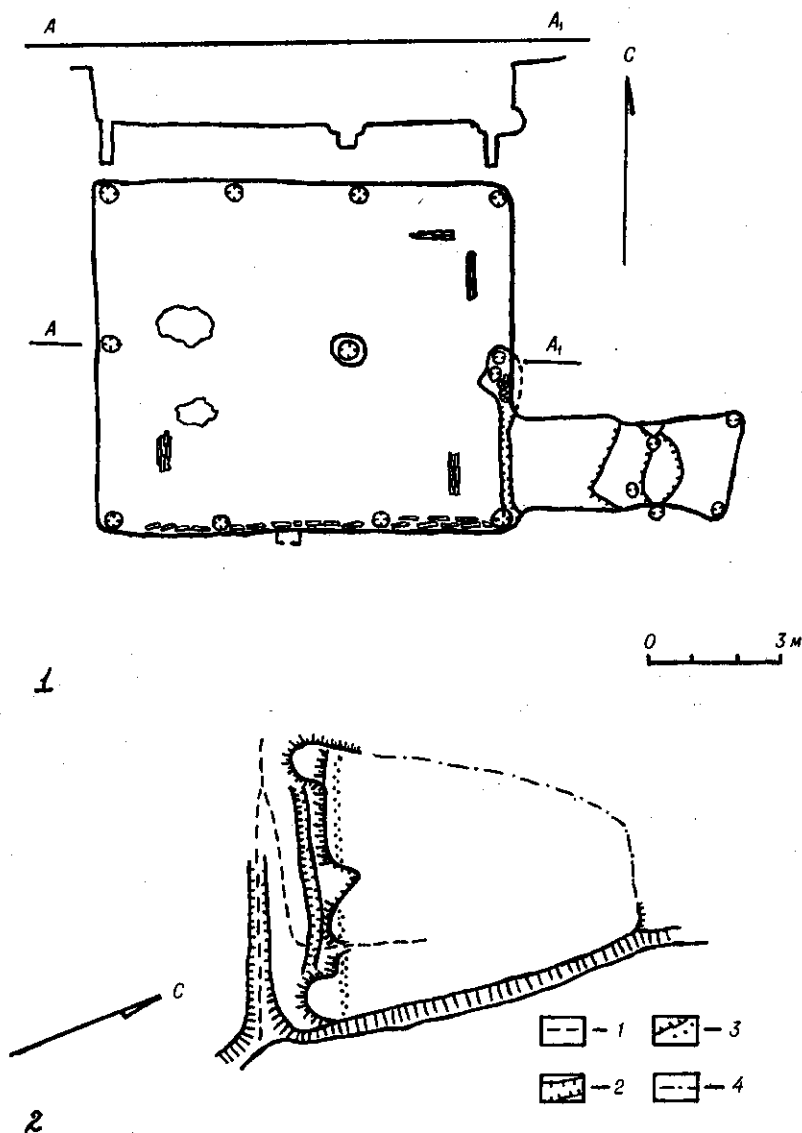
Рис. 3. 1 — План і розріз куреня; 2 — План городища біля оз. Підкручного (о. Хортиця).
