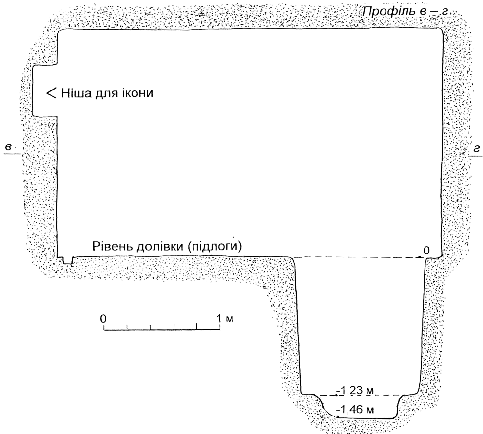
Рис. 4. Печера біля с. Велика Воля. Профіль в-г
