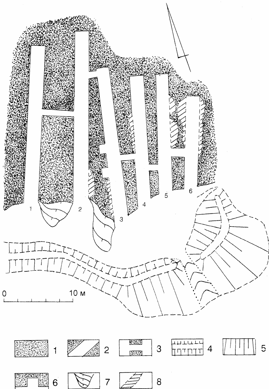
Рис. 17. План печерного комплексу III: 1 – скеля; 2 – зала; 3 – прохід; 4 – земляний вал; 5 – схили; 6 – ніша; 7 – скельний виступ, 8 – поруйновані частини комплексу Fig. 17. Plan of cave complex III: 1 – rock; 2 – hall; 3 – entrance; 4 – earthen billow; 5 – slopes; 6 – niche; 7 – rock ledge; 8 – ruined part of the complex
