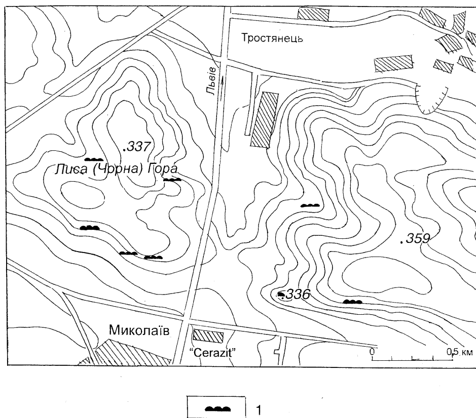
Рис. 9. План-схема розташування печерних комплексів на околиці м. Миколаєва в ур. Лиса (Чорна) Гора
