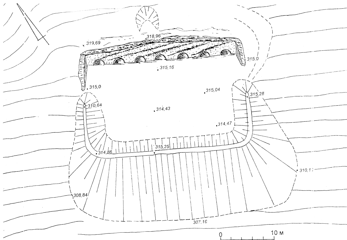
Рис. 10. Миколаїв, ур. Лиса (Чорна) Гора. Геодезичний план печерного комплексу I
