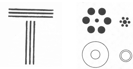
Рис. 7. Деякі оптико-геометричні ілюзії сприйняття
