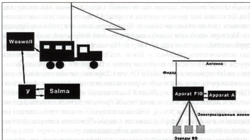
Схема під'єднання об'єктних мін F-10 (радіоміні)
