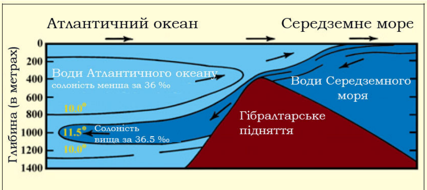
Мал. 13. Води Середземного моря досягають Атлантичного океану над Гібралтарським підняттям, зберігаючи власну температуру, солоність і густину внаслідок того, що “перепона” відділяє їх від вод Атлантики. Температура за Цельсієм (Marine Geology, Kuennen, p. 43, з деякими доповненнями.)
