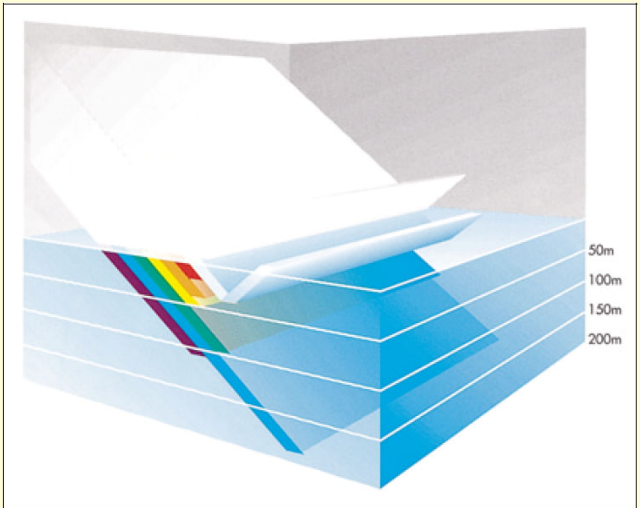
Мал. 15. Від 3 до 30 відсотків сонячного світла заломлюється на поверхні моря. Майже всі сім кольорів світлового спектру поглинаються один за іншим, ледь досягаючи глибини в 200 м., окрім синього кольору. (Oceans, Elder and Pernetta, p. 27.)
