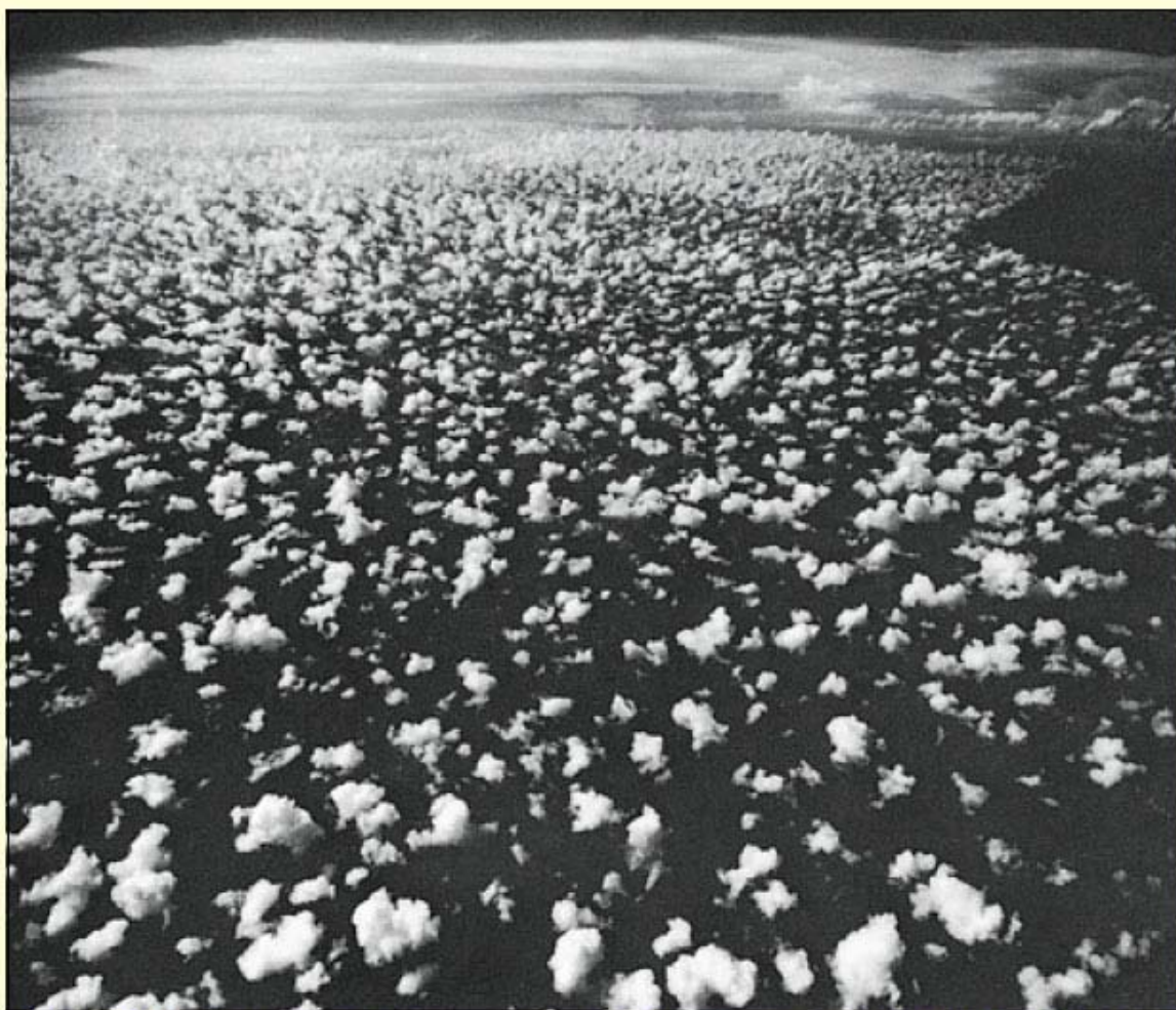
Мал. 18. Маленькі частинки хмар (купчасті хмари) рухаються в напрямі зони скупчення біля обрію, де ми можемо бачити велику дощову хмару. (Clouds and Storms, Ludlam, plate 7.4.)
