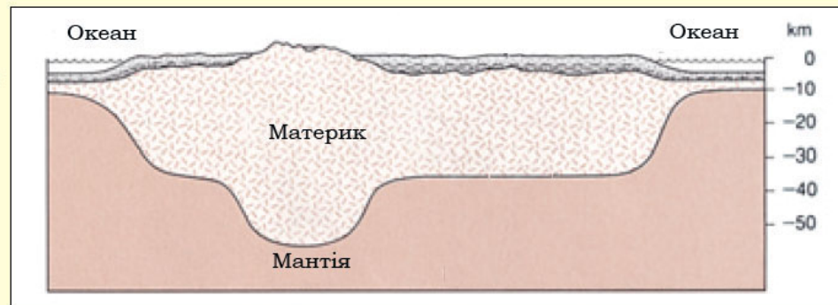
Мал. 7. Корені гір досягають великих глибин під поверхнею землі (Earth, Press and Siever, p. 413.)
