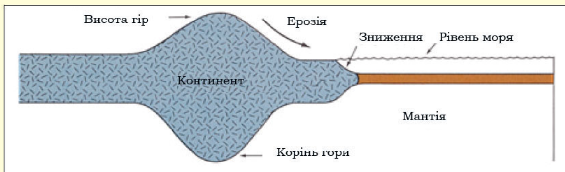
Мал. 9. Інша ілюстрація демонструє, як гори схожі на кілки через свої глибокі корені. (Earth Science, Tarbuck and Lutgens, p. 158.)
