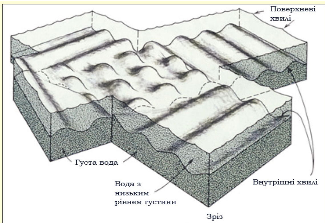
Мал. 16. Внутрішні хвилі виникають між двома шарами води з різними рівнями густини (вищим і нижчим). (Oceanography, Gross, p. 204.)
