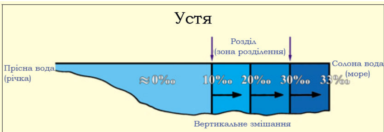
Мал. 14. Повздовжній розріз показує рівень солоності (тисячні ‰) в усті. Ми спостерігаємо розділ (зону розділення) між прісною і солоною водою. (Introductory Oceanography, Thurman, p. 301, з деякими доповненнями.)
