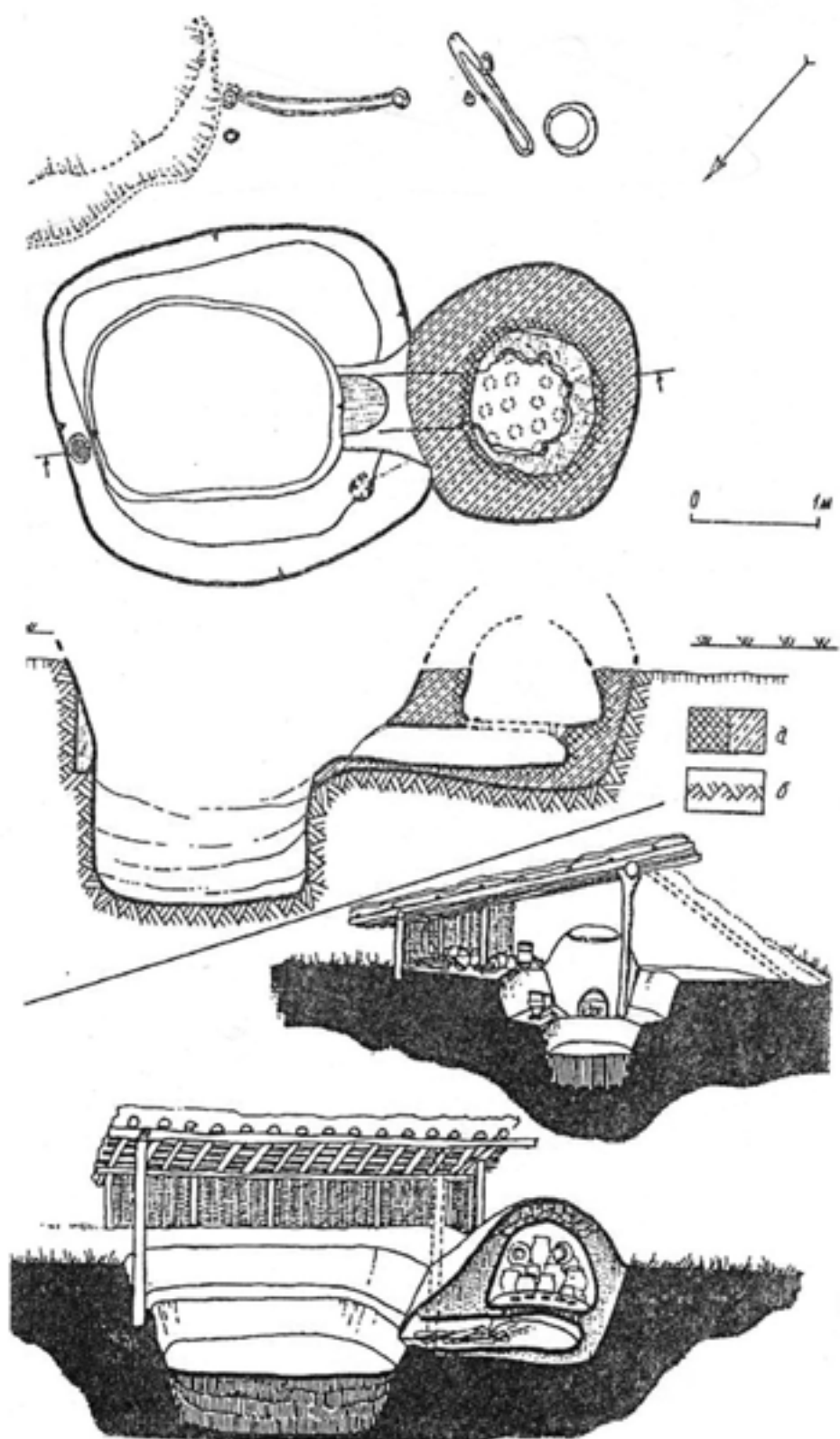
Рис. 23. Гончарне горно № 6 з поселення Автуничі за автором, Т.Г. Новик і П.Л. Корнієнком.
