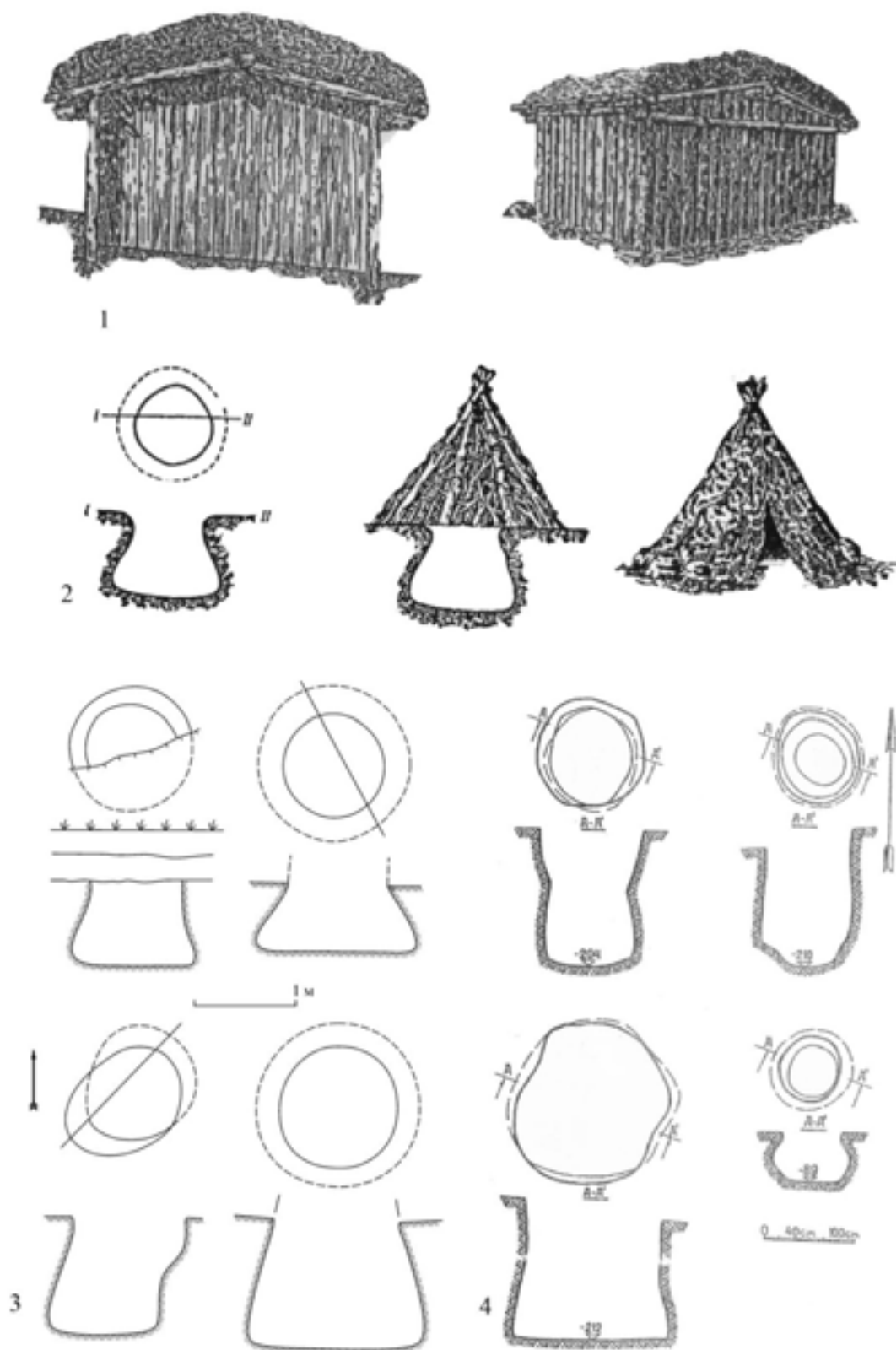
Рис. 38. Господарські споруди (1) і ями для припасів з гаданим зовнішнім виглядом їх перекриття (2) з Новотроїцького за І. І. Ляпушкіним та ями для збіжжя з поселень Ходосівка-Козаків яр (3) і Гульськ (4).
