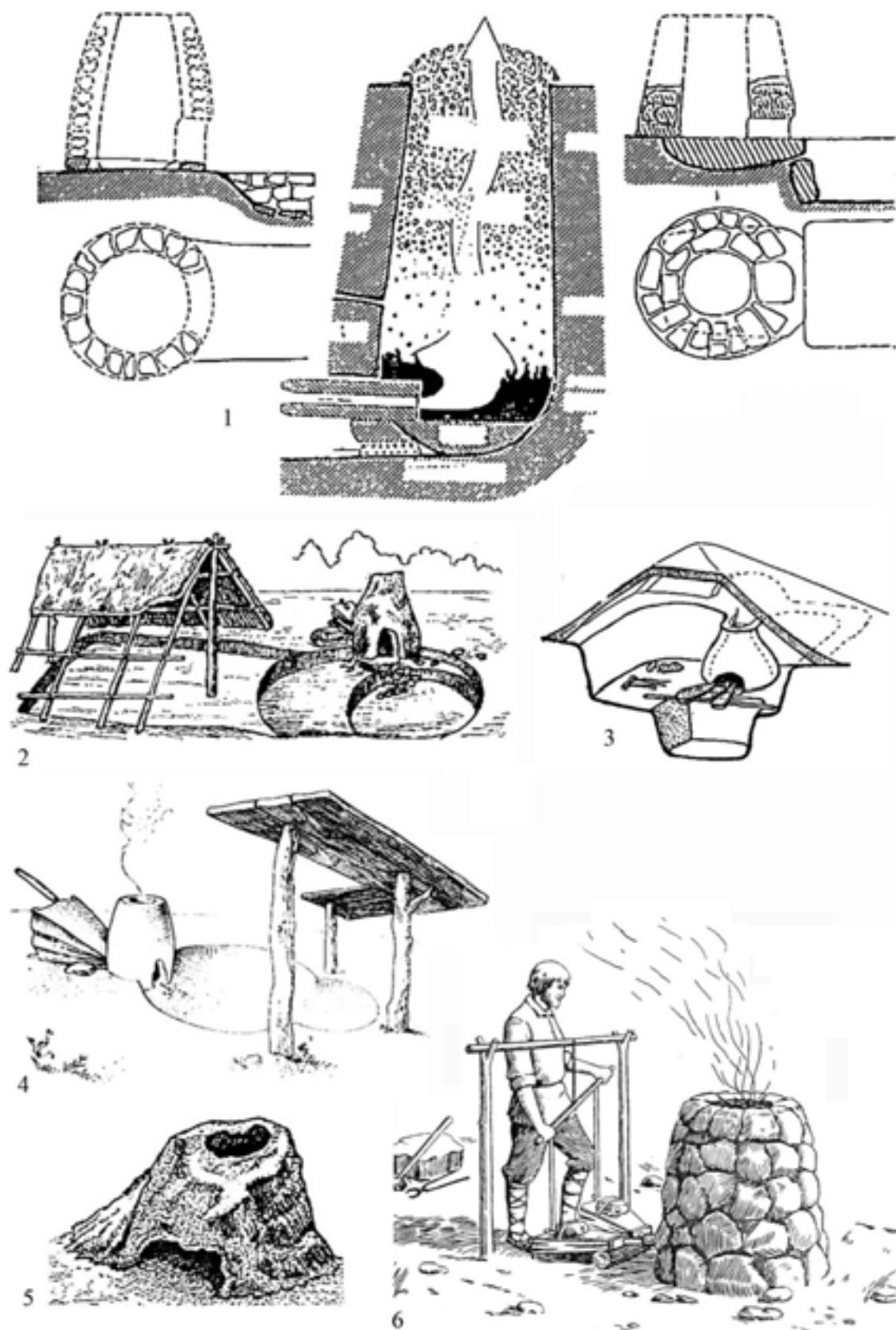
Рис. 29. Схема влаштування залізоборних споруд за Б.О. Колчиним (1) та гаданий зовнішній вигляд об'єктів чорнометалургійної галузі із слов'яно-руських пам'яток за Б.О. Колчиним (1, 3, 6), В.І. Бідзілею (2), В.І. Бідзілею, Г.О. Вознесенською, Д.П. Недопако, С.В. Паньковим (4) та В.В. Седовим (5).
