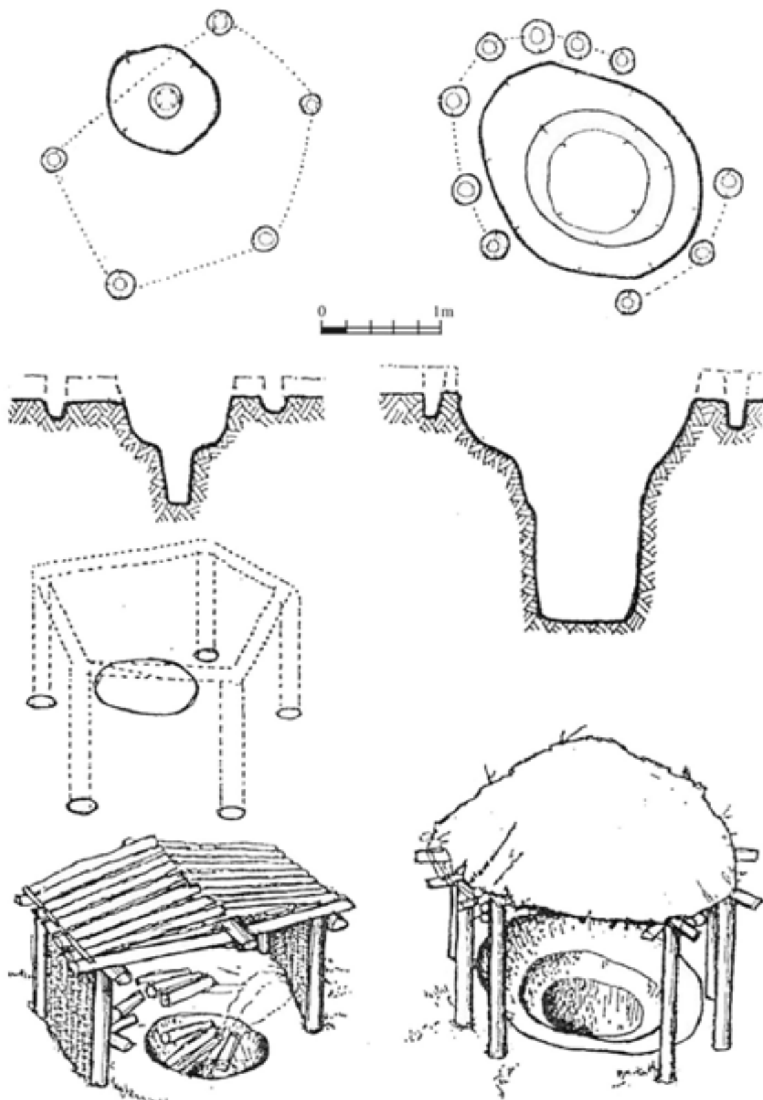
Рис. 33. Споруди для ямного смолокуріння і дигтярства з Автуничів за автором, Т.Г. Новик і П.Л. Корнієнко.
