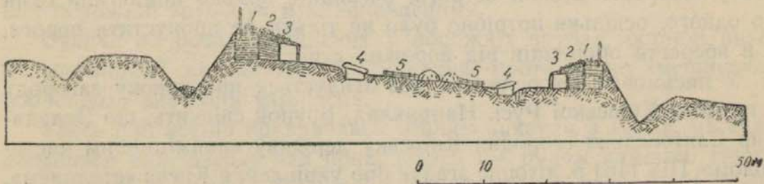
Рис. 14. План і розріз оборонних споруд Райковецького городища (Бердичівський район, Житомирської області), розкопаного в 1928—1937 рр. 1 — тараси; 2 — житлові кліті; 3 — господарські кліті; 4 — землянки; 5 — місця загород для худоби.
