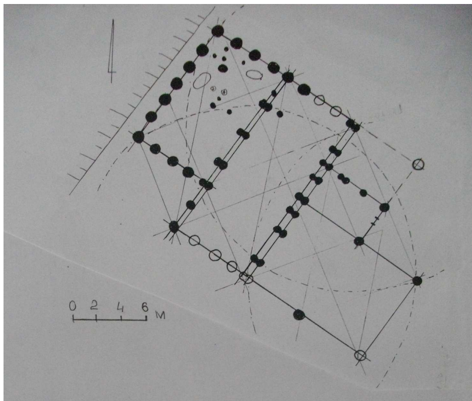
Рис.5. Крилоське городище. Княжий двір. Західний палацовий комплекс (XII – XIII ст.)
