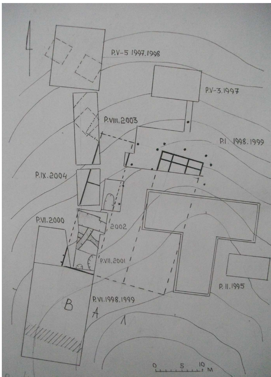
Рис.4. Крилоське городище. Південний палацовий комплекс. Перший будівельний горизонт (середина XII ст.)
