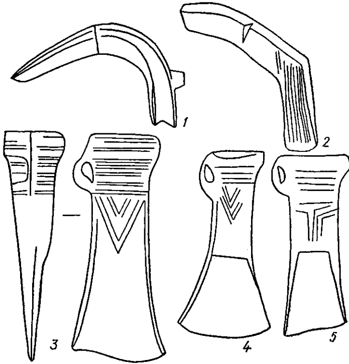
Рис. 10. Горизонт Мойград-Теутеу.
