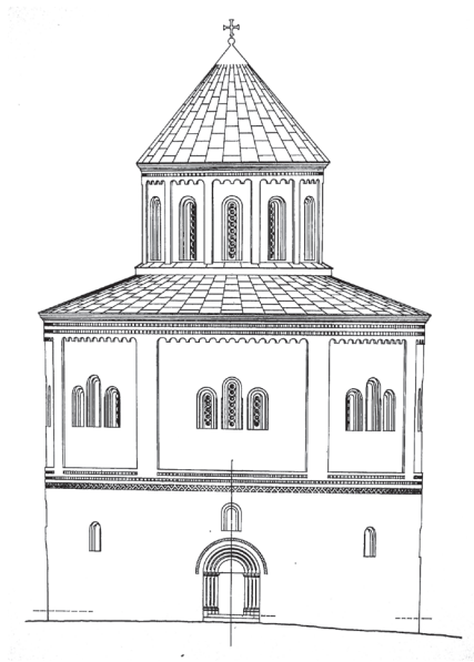
Ротонда архангела Михаїла у Володимирі. Реконструкція Ю. Діби
