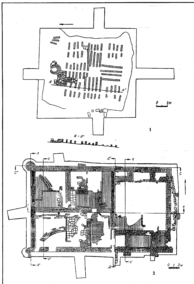
Рис. 5. Планы обогревательной системы бани (1) и «резиденции феодала» (2) городища Большие Кучугуры.
