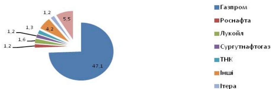
Рис. 7. Обсяги видобутку природного газу російськими компаніями у 2012 р. (кбк/добу) [10]
