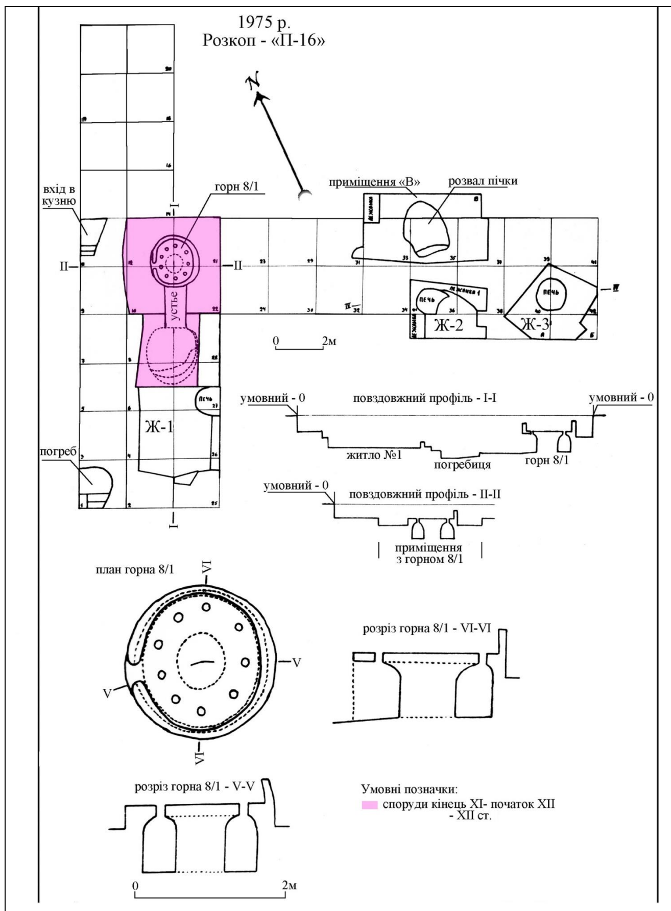
Рис. 59. План та розрізи гончарного горна рубежу XI-XII—XII ст.
