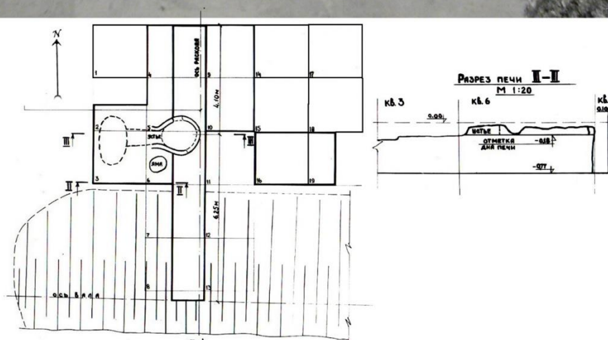
Рис. 70. «Металургійний» горн розкопаний поблизу поперечного валу посаду. (за Є.А. Ліньовою)
