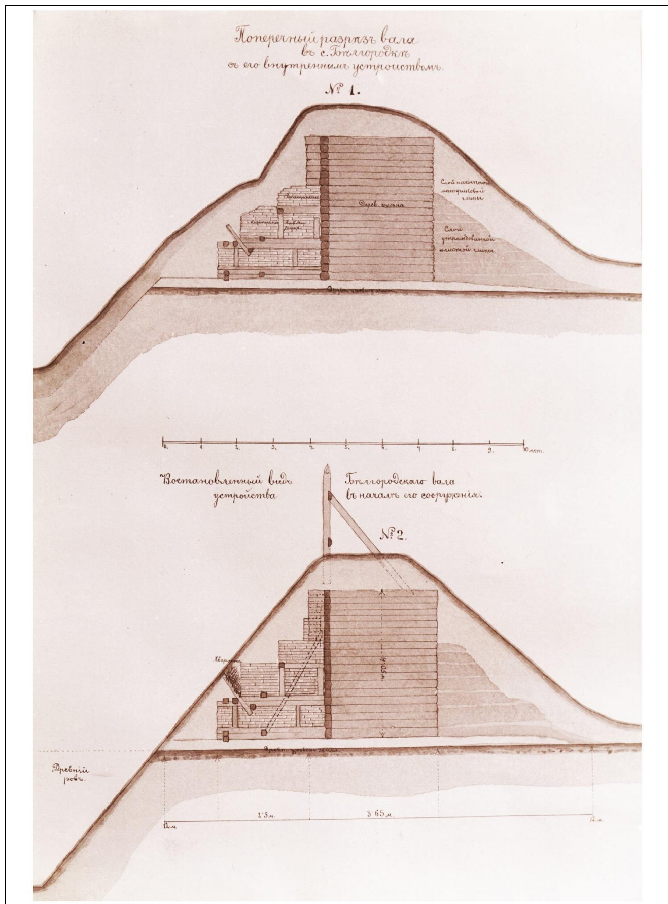
Рис. 12. Креслення розрізу валу посаду. (за В.В. Хвойко)
