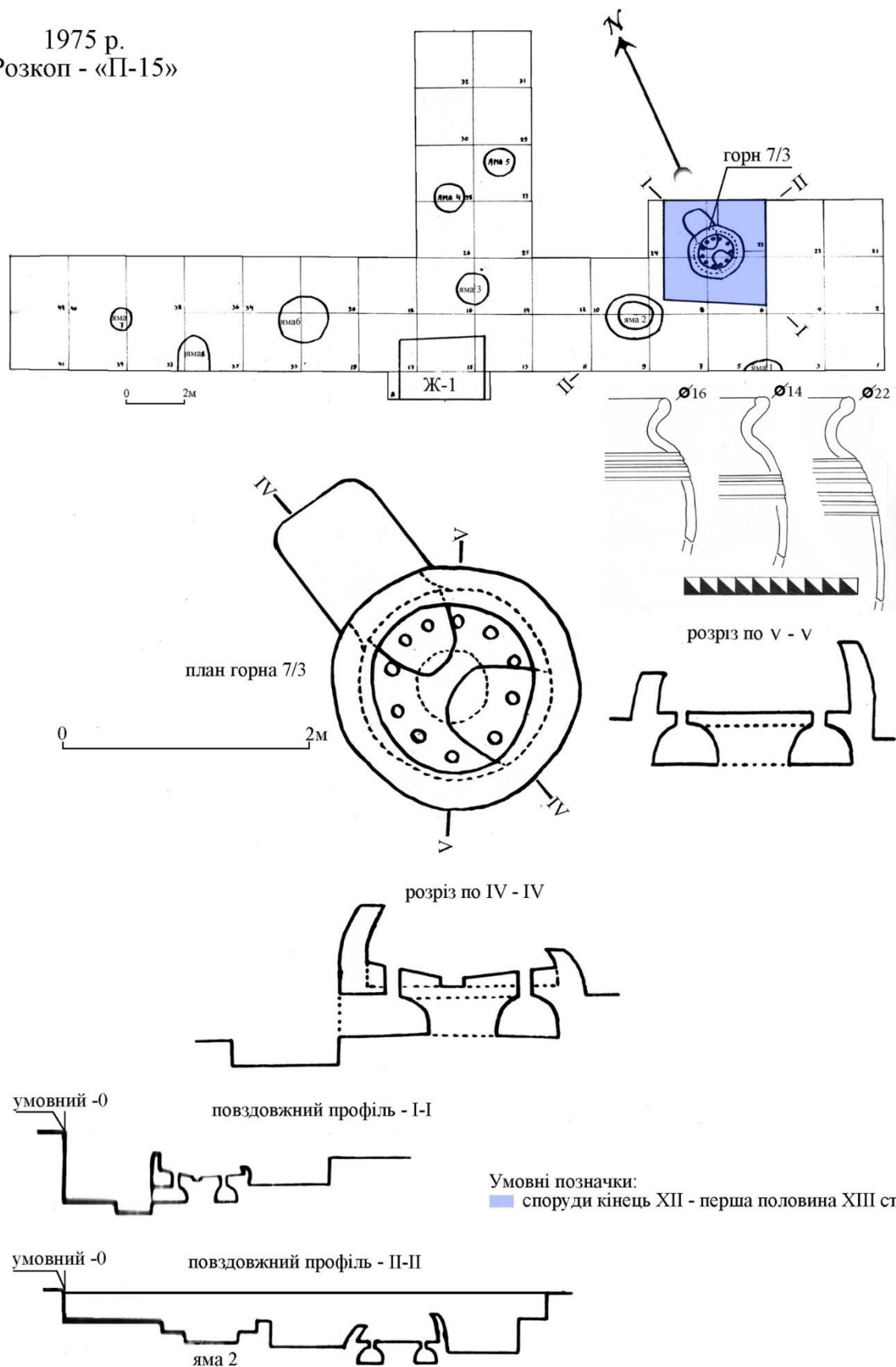
Рис. 68. План та профілі розрізів гончарного горна кінця XII — першої половини XIII ст. дослідженого Г.Г. Мезенцевою.
