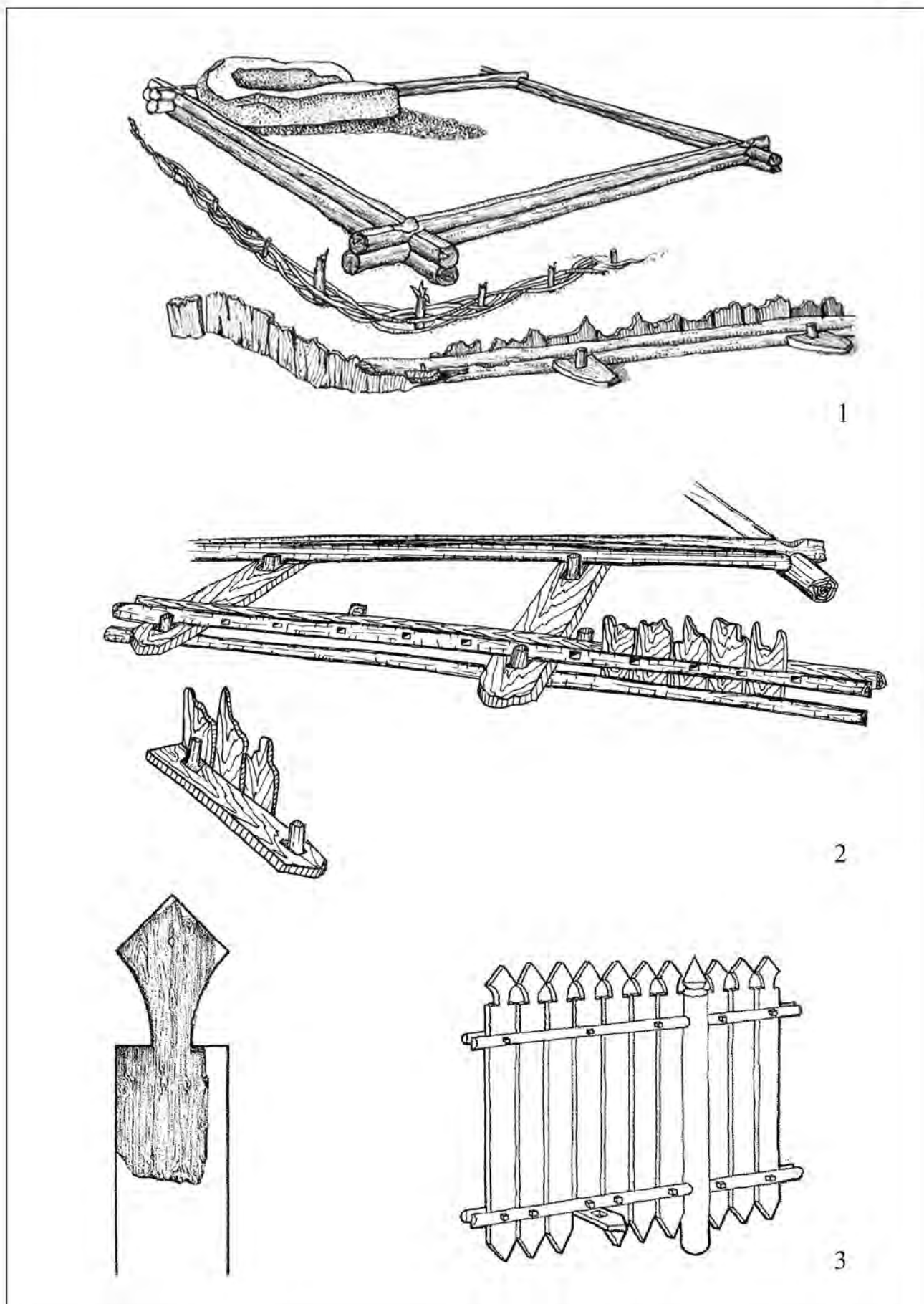
Рис. 30. Конструкція укріплення паркану біля зрубу 1 в садибі В на Житньому ринку київського Подолу (1, 2) та реконструкція В.О. Харламова подільського дощатого паркану (3) (матеріали В.О. Харламова та [Харламов, 1976, с. 53, рис. 9]).
