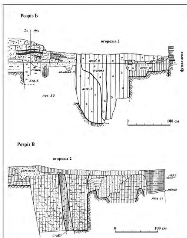
Рис. 28. Дерев'яна огорожа-стовп'я початку XII ст. (огорожа 1) та кінця XII ст. (огорожа 2) Михайлівського Золотоверхого монастиря в Києві. План (1), розрізи (2) та фото (3) огорожі за [Козюба, 2010а, с. 46-48, рис. 2-4].
