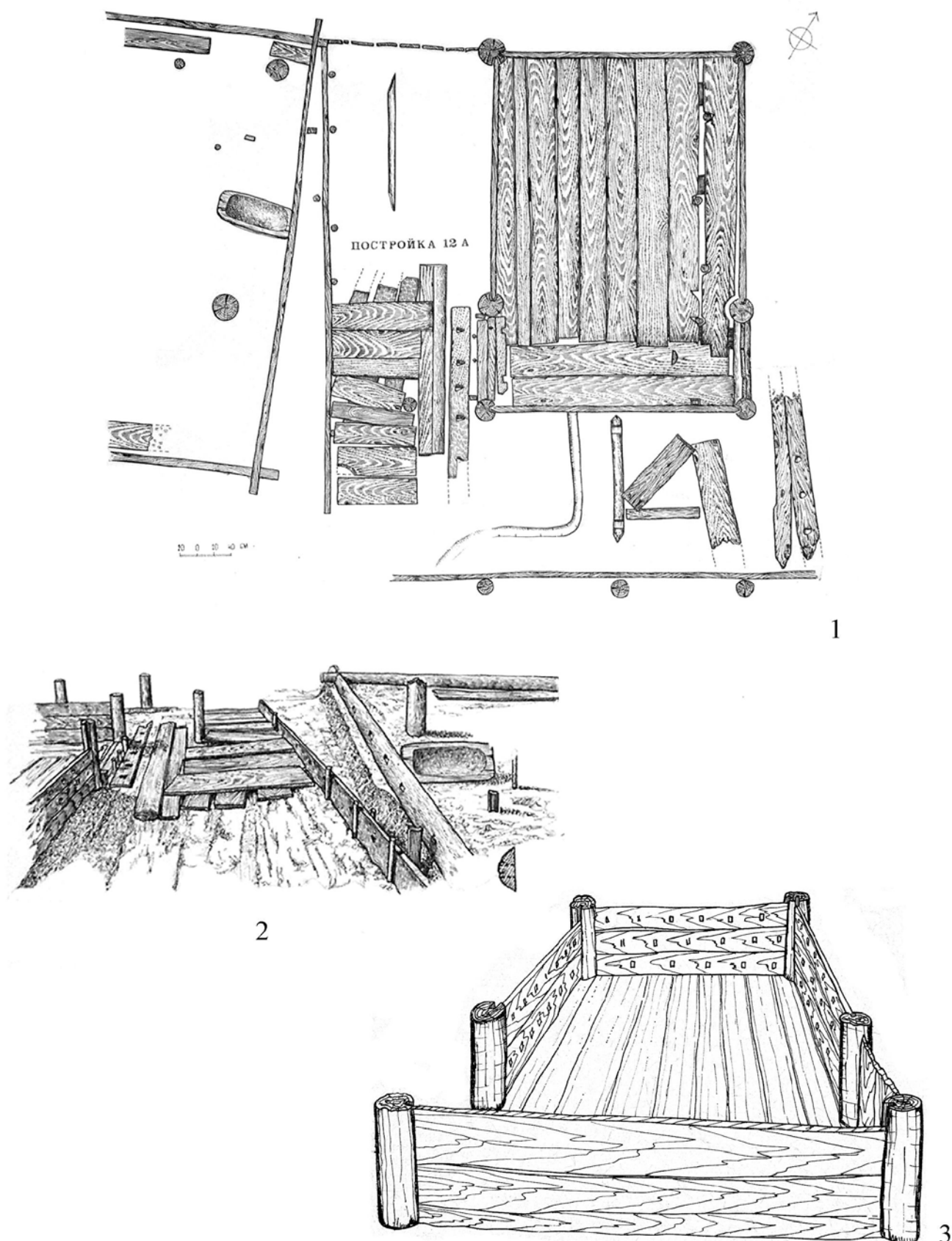
Рис. 22. План споруд 12 та 12А в садбі В на Житньому ринку київського Подолу (1), малюнок помосту між ними (2) (матеріали В.О. Харламова), виробнича споруда 12А (3) за [Харламов, 1976, с. 51, рис. 30].
