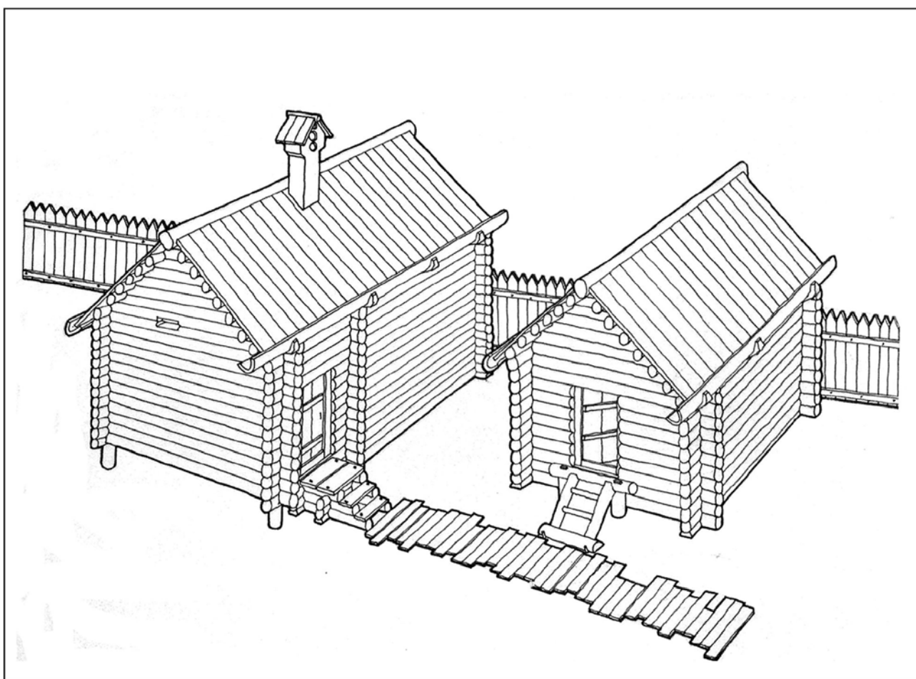
Рис. 39. Зруби 7, 8 садиби В на Житньому ринку за [Харламов, 1981, с. 128, рис. 46] та їх реконструкція В.О. Харламова
