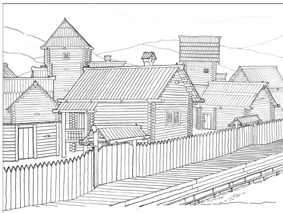
Рис. 15. Льох Х ст. в садибі В на Житньому ринку (1) та реконструкція забудови подільських садиб у Києві (2) за матеріалами В.О. Харламова.
