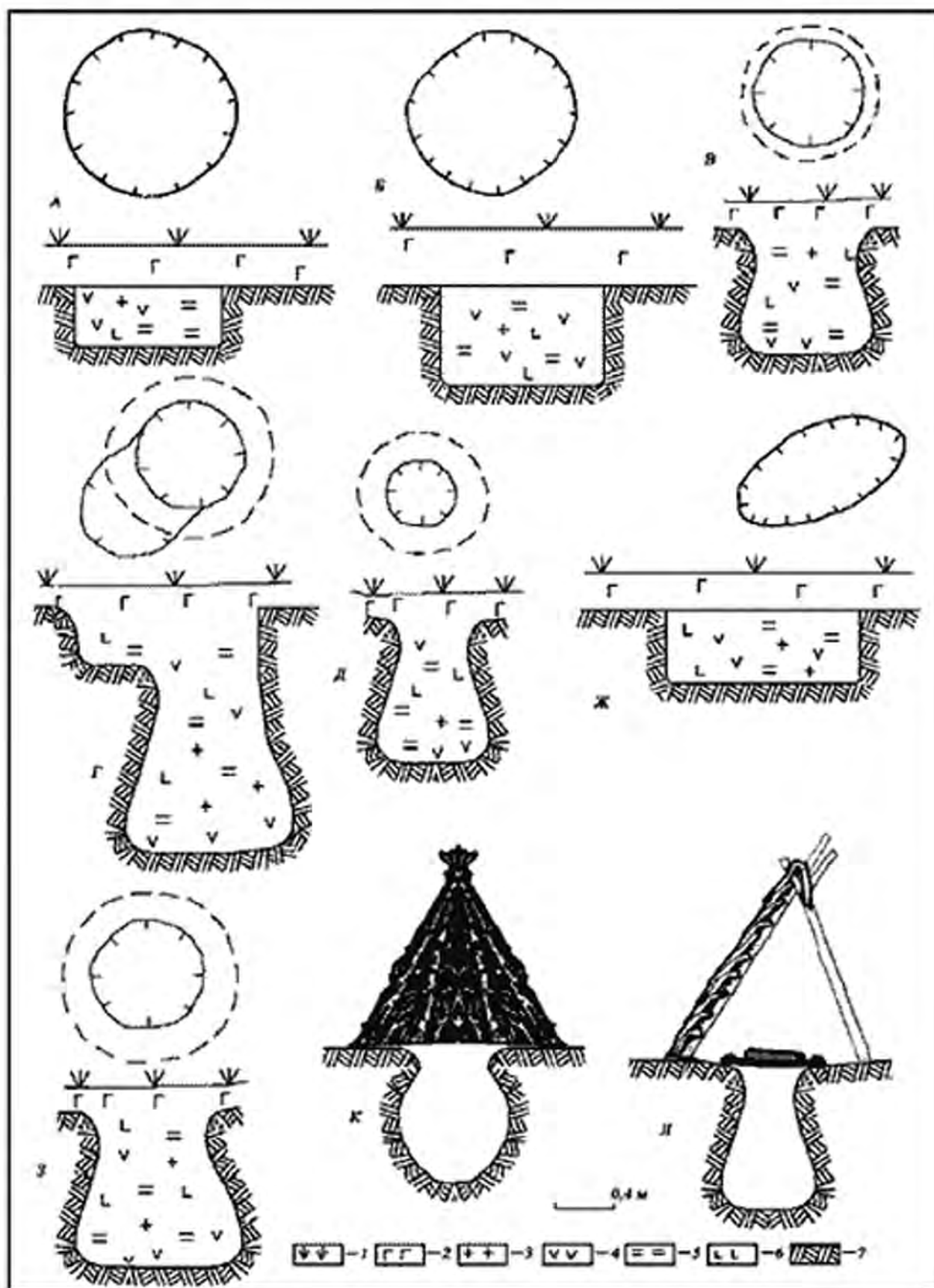
Рис. 14. Господарські ями з поселень Сіreto-Дністровського межириччя за [Возний, 2009, с. 173, рис. 1].
