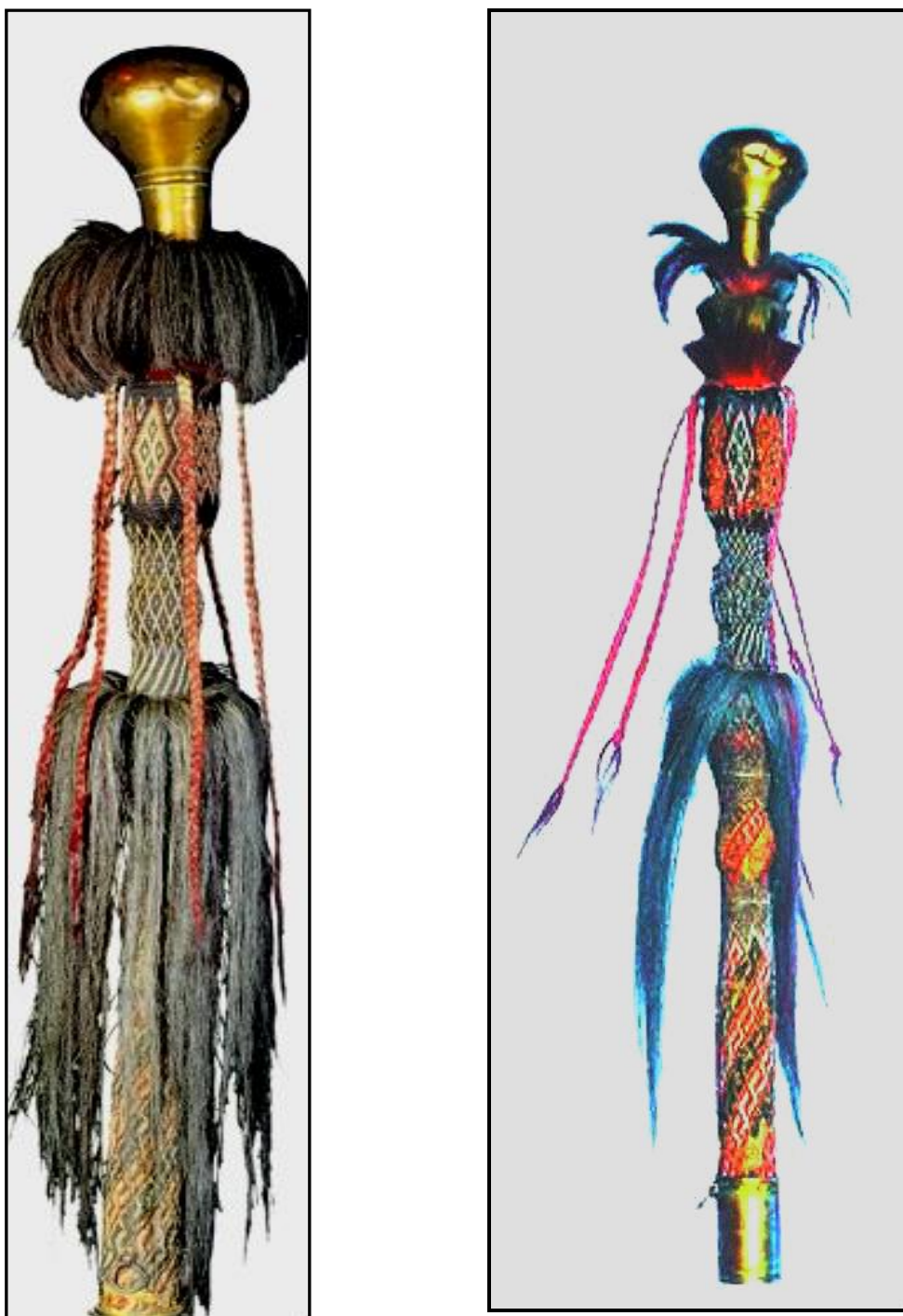
Рис. 19. Бунчуки XVII ст. Из колекції НМІУ та ХОКМ [447, с. 523]
